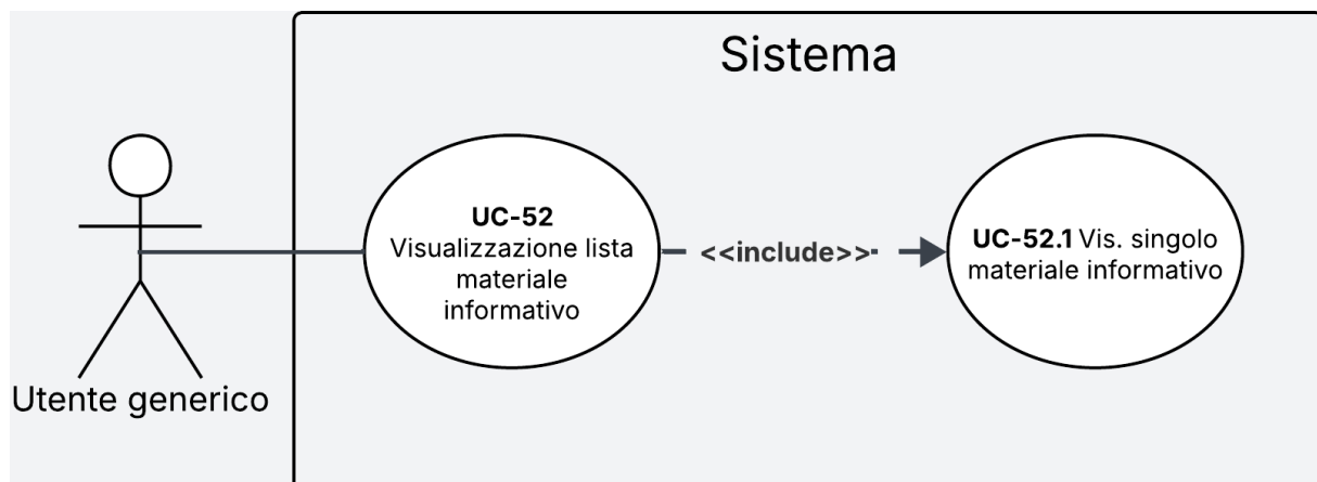
Figura 36: Diagramma del caso d'uso UC-52
