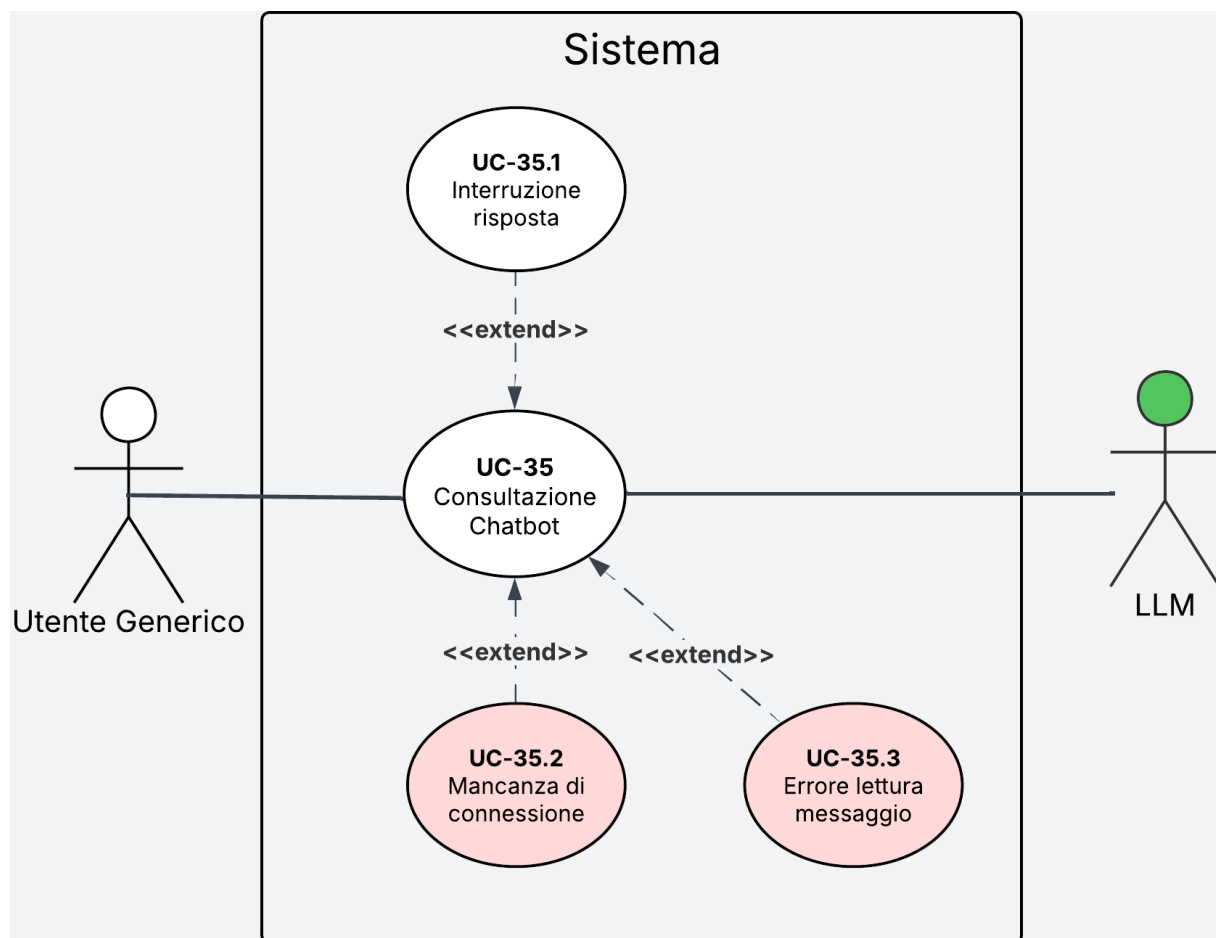
Figura 24: Diagramma del caso d'uso UC-35
