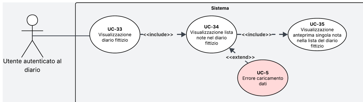
Figura 22: Diagramma del caso d'uso UC-33
