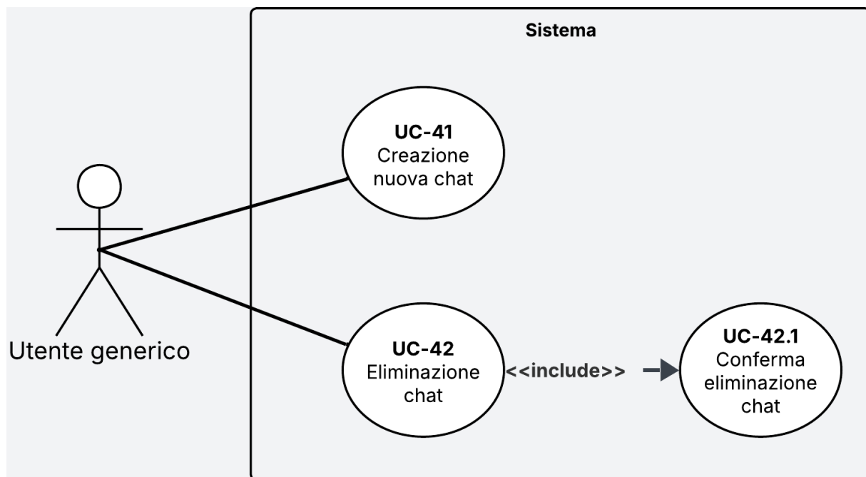
Figura 29: Diagramma dei casi d'uso UC-41 e UC-42
