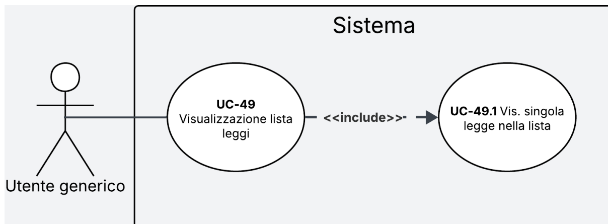
Figura 34: Diagramma del caso d'uso UC-49
