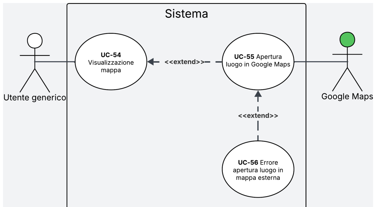
Figura 38: Diagramma del caso d'uso UC-54
