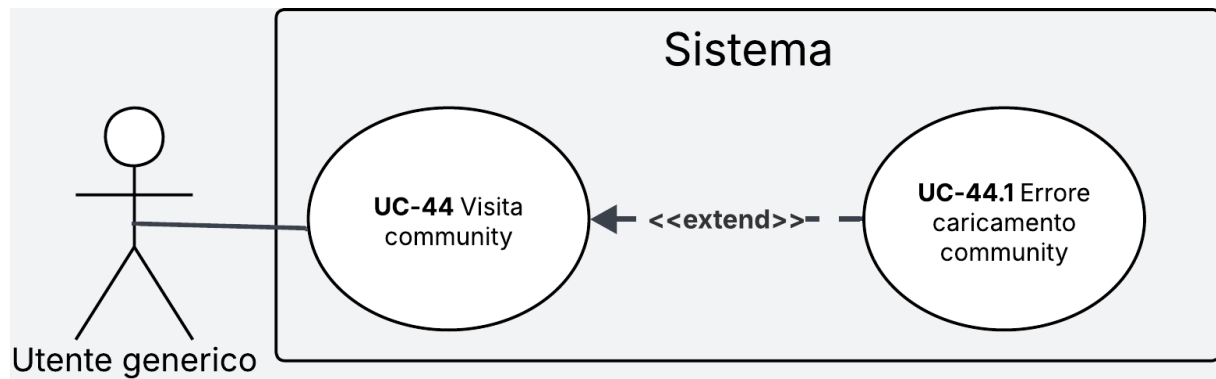
Figura 31: Diagramma del caso d'uso UC-44
