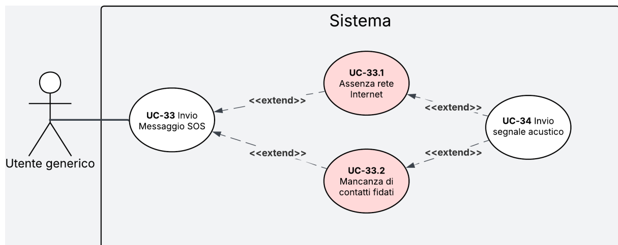
Figura 23: Diagramma del caso d'uso UC-33
