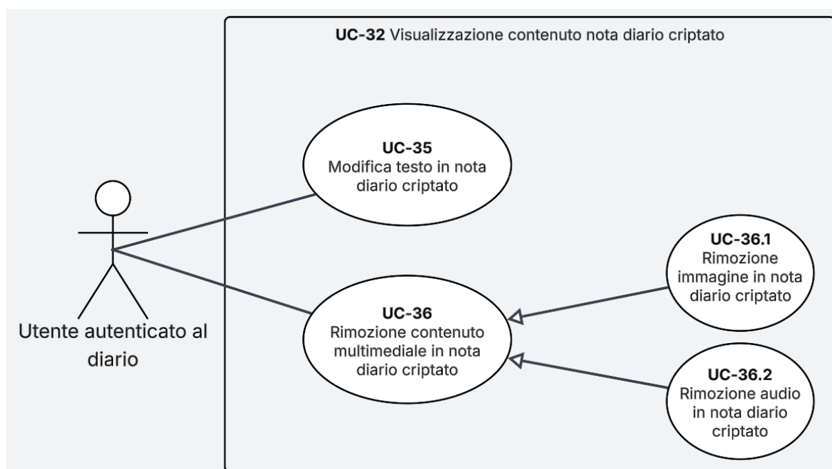
Figura 21: Diagramma dei casi d'uso UC-35, UC-36, UC-36.1 e UC-36.2
