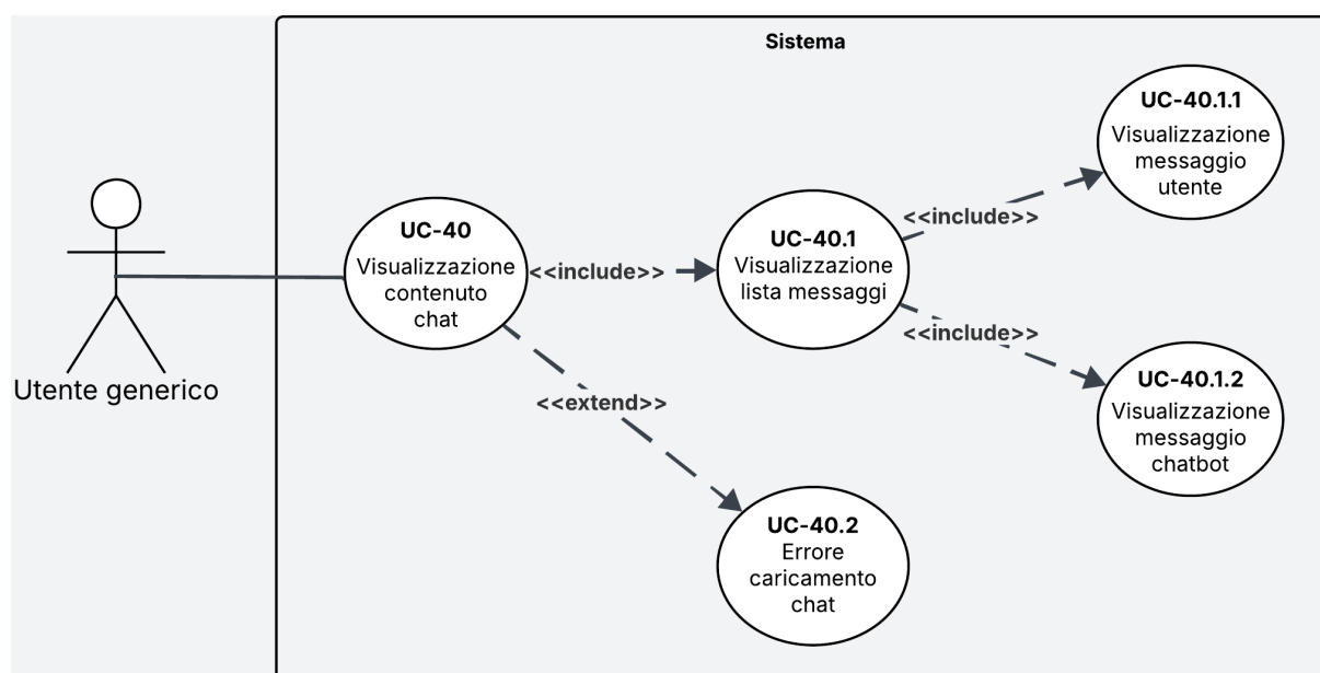
Figura 28: Diagramma del caso d'uso UC-40
