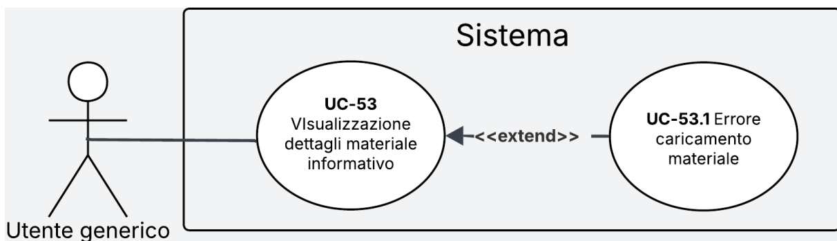
Figura 37: Diagramma del caso d'uso UC-53
