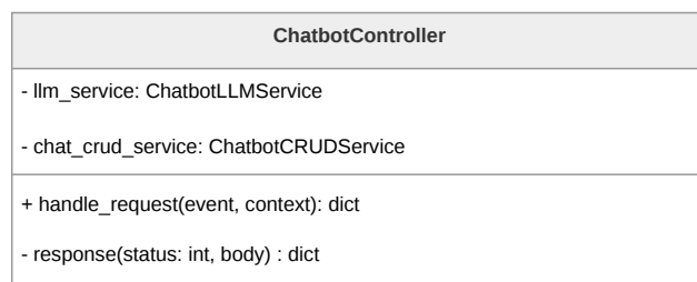
Figura 180: Diagramma della classe ChatBotController
