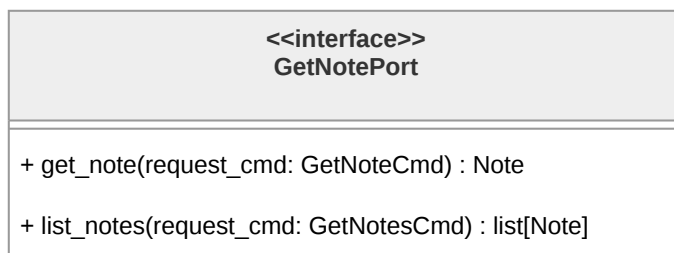
Figura 139: Diagramma dell'interfaccia GetNotePort
