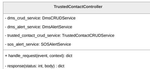
Figura 192: Diagramma della classe TrustedContactController
