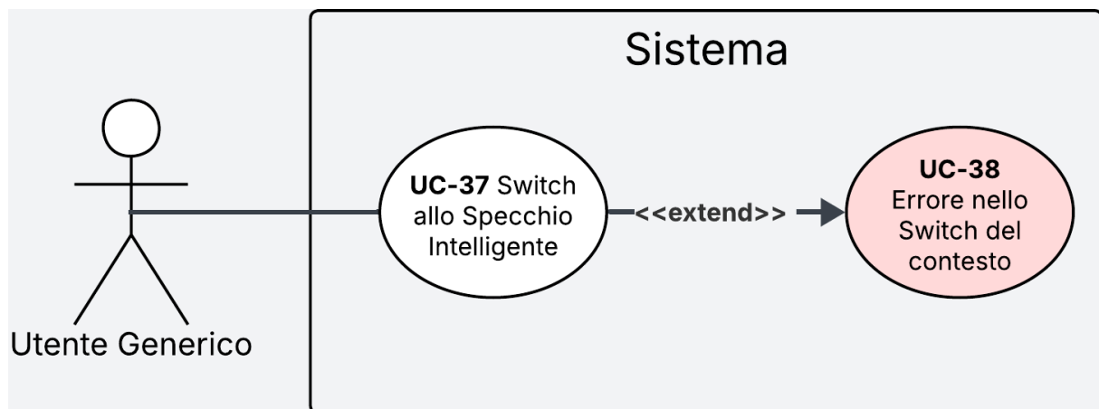
Figura 26: Diagramma del caso d'uso UC-37
