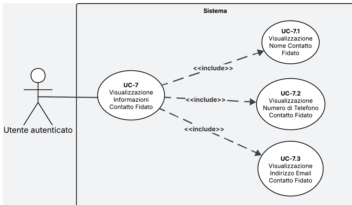
Figura 5: Diagramma del caso d'uso UC-7
