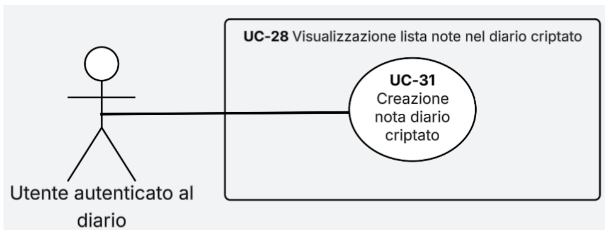
Figura 20: Diagramma del caso d'uso UC-31
