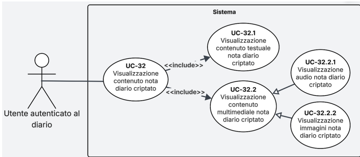
Figura 22: Diagramma del caso d'uso UC-32
