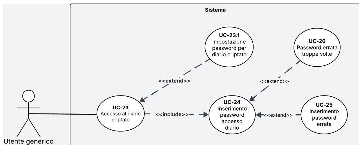
Figura 15: Diagramma del caso d'uso UC-23
