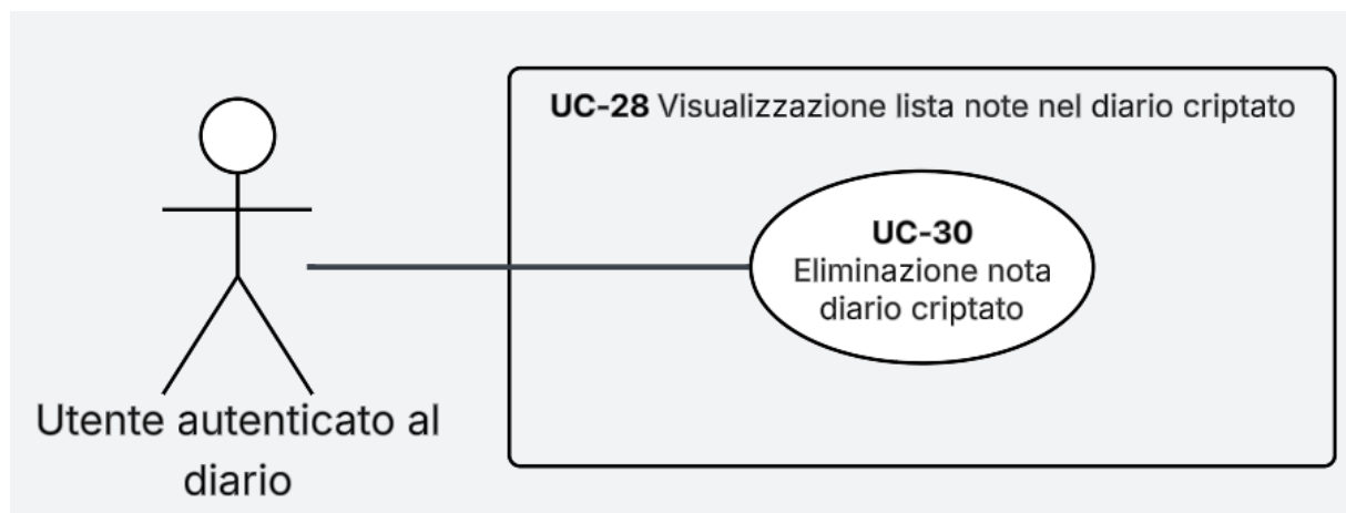
Figura 18: Diagramma del caso d'uso UC-30
