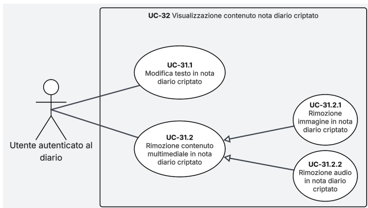
Figura 21: Diagramma dei casi d'uso UC-31.1, UC-31.2, UC-31.2.1 e UC-31.2.2
