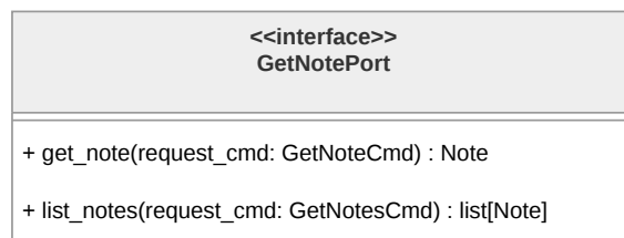
Figura 209: Diagramma dell'interfaccia GetNotePort
