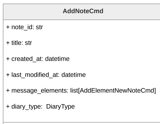
Figura 202: Diagramma della classe AddNoteCmd
