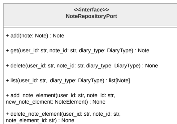
Figura 217: Diagramma dell'interfaccia NoteRepositoryPort
