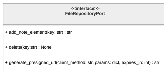
Figura 218: Diagramma dell'interfaccia FileRepositoryPort
