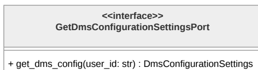
Figura 179: Diagramma della classe GetDmsConfigurationSettingsPort
