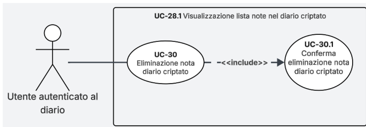
Figura 17: Diagramma dei casi d'uso UC-30 e UC-30.1
