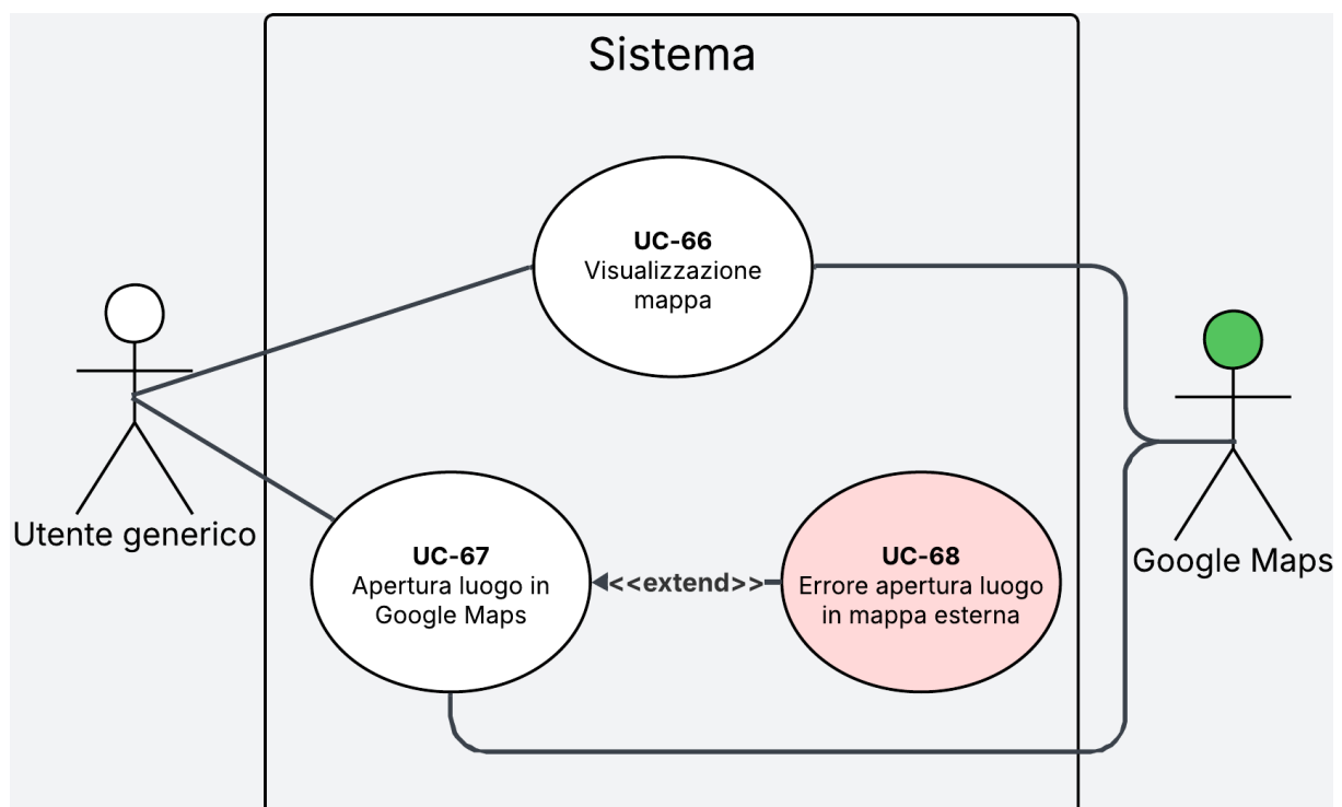
Figura 43: Diagramma dei casi d'uso UC-66 e UC-67
