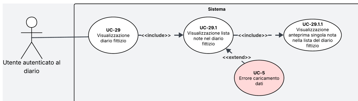
Figura 22: Diagramma del caso d'uso UC-29
