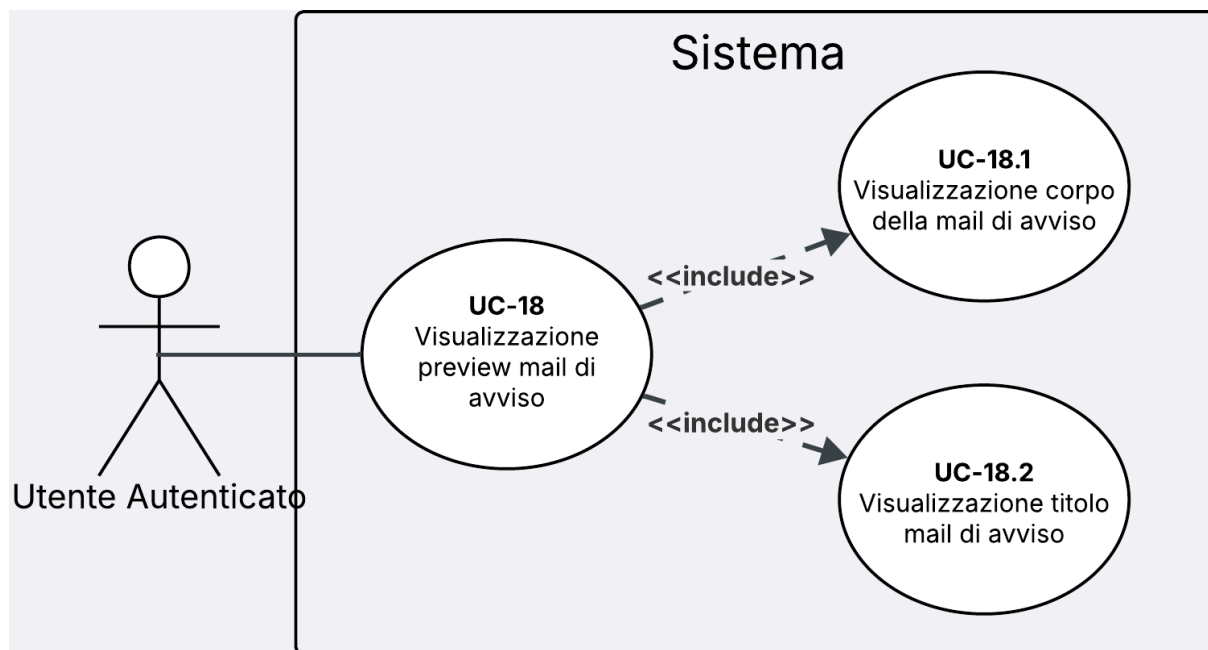
Figura 12: Diagramma del caso d'uso UC-18
