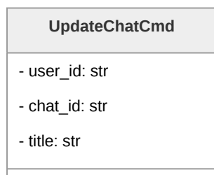
Figura 195: Diagramma della classe UpdateChatCmd
