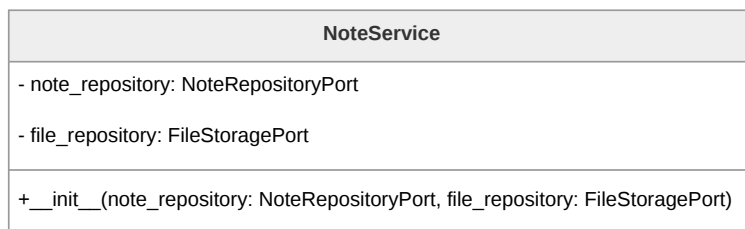
Figura 168: Diagramma della classe NoteService
