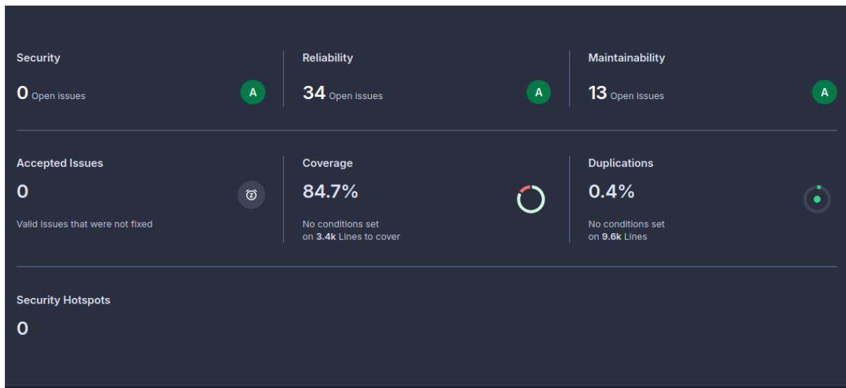
Figura 11: Cruscotto metriche codice frontend
