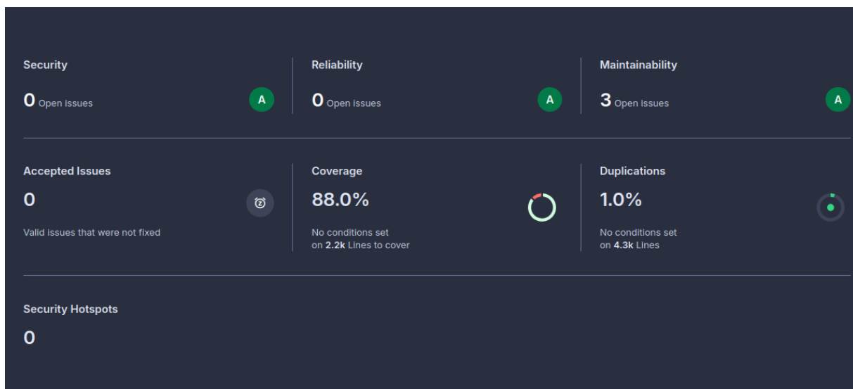
Figura 12: Cruscotto metriche codice backend
