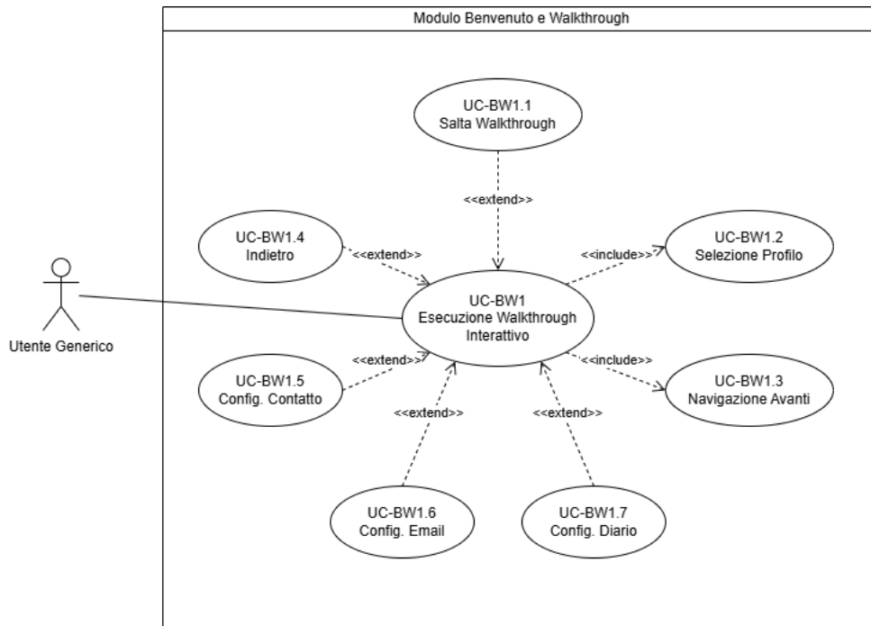
Figura 1: Diagramma del caso d'uso UC-BW1
