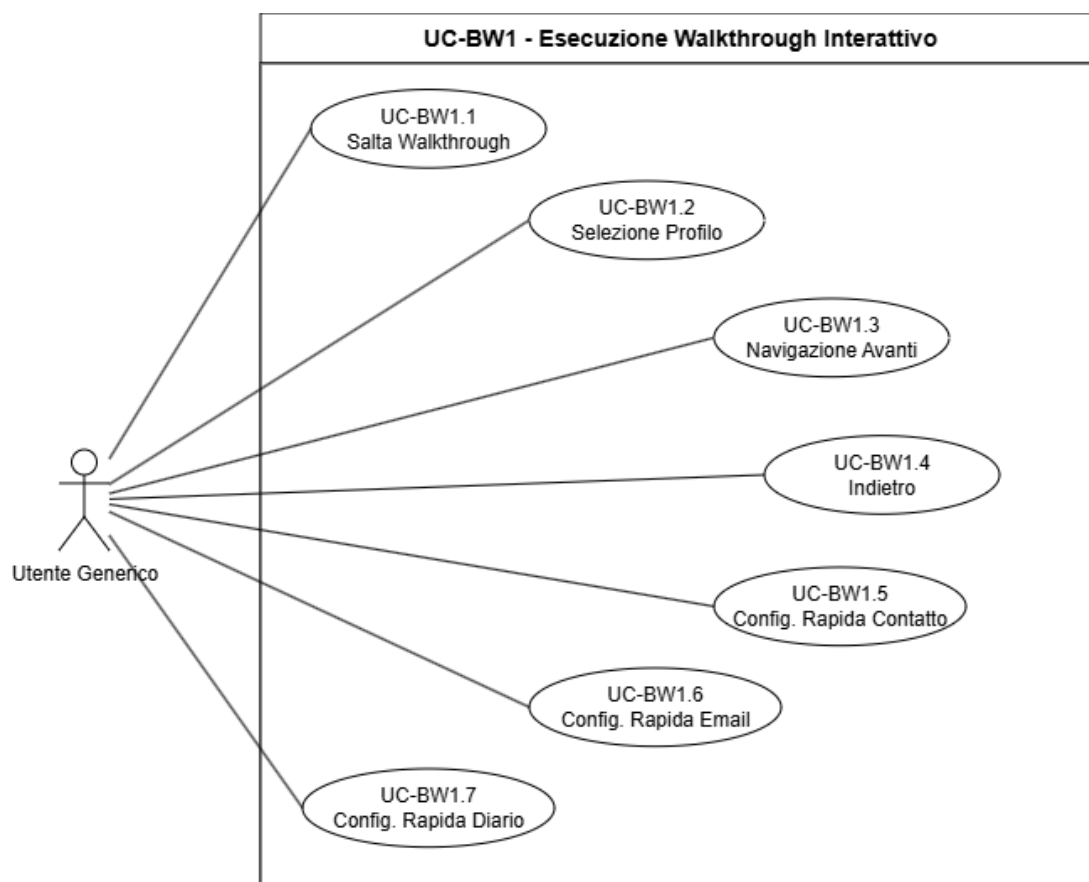
Figura 2: Dettaglio inclusioni ed estensioni del caso d'uso UC-BW1
