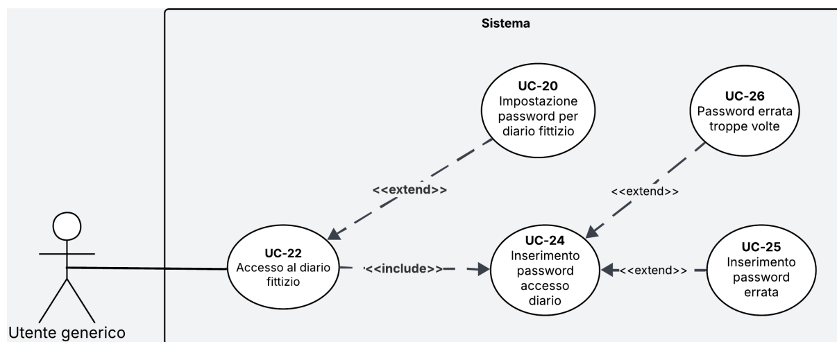
Figura 14: Diagramma del caso d'uso UC-22
