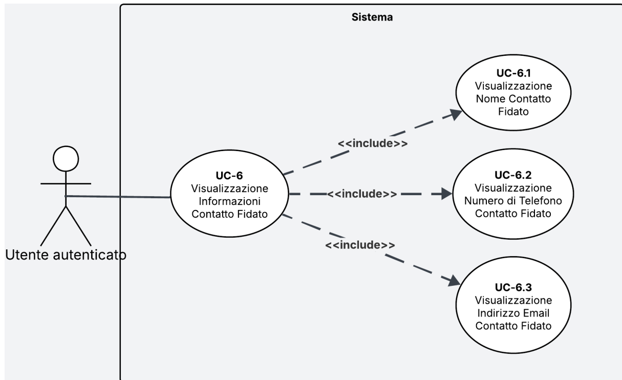
Figura 5: Diagramma del caso d'uso UC-6 con relativi sottocasi d'uso
