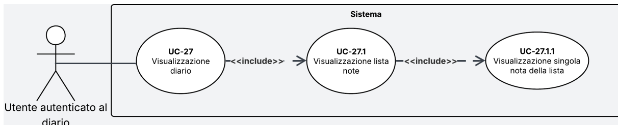
Figura 17: Diagramma del caso d'uso UC-27
