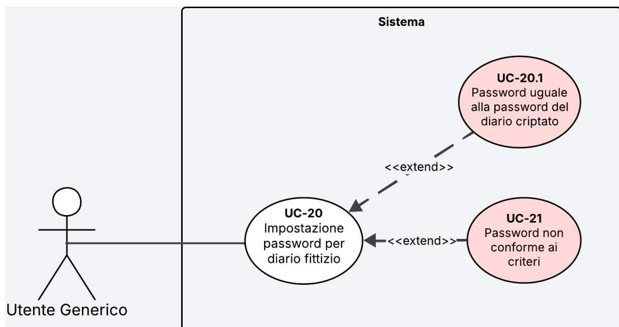
Figura 13: Diagramma del caso d'uso UC-20
