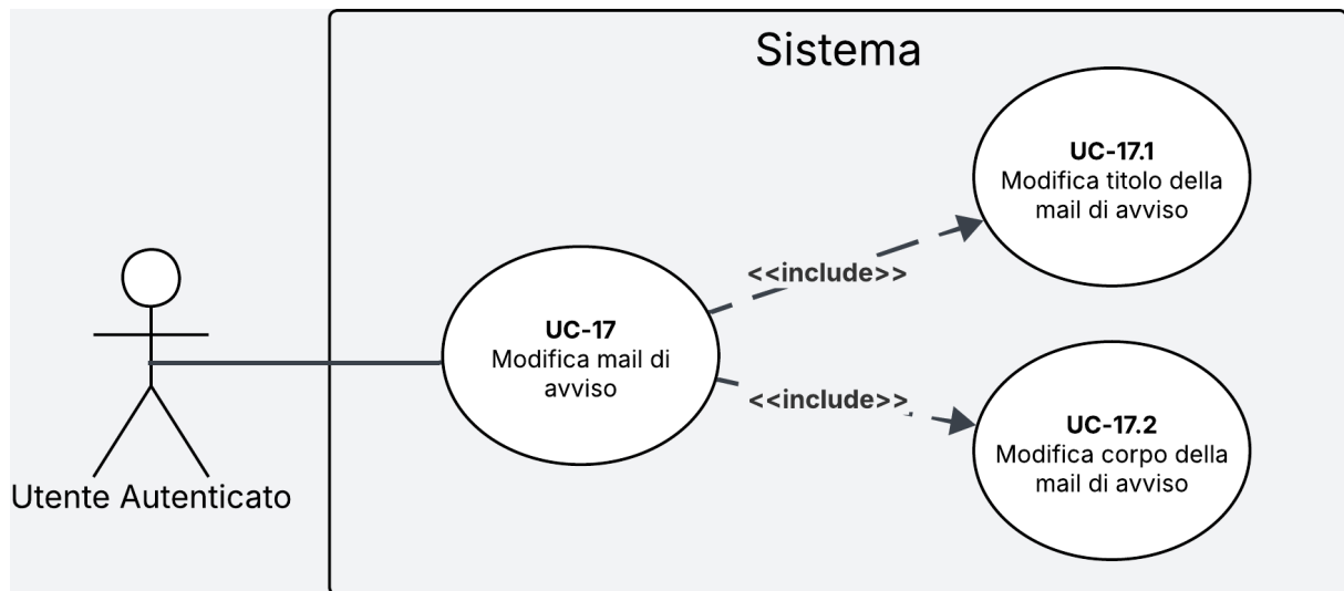
Figura 10: Diagramma del caso d'uso UC-17
