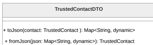
Figura 68: Diagramma della classe TrustedContactDTO
