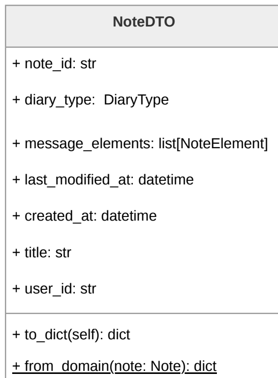
Figura 147: Diagramma della classe NoteDTO
