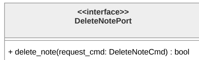
Figura 141: Diagramma dell'interfaccia DeleteNotePort
