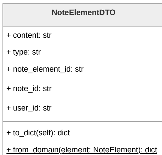
Figura 172: Diagramma della classe NoteElementDTO
