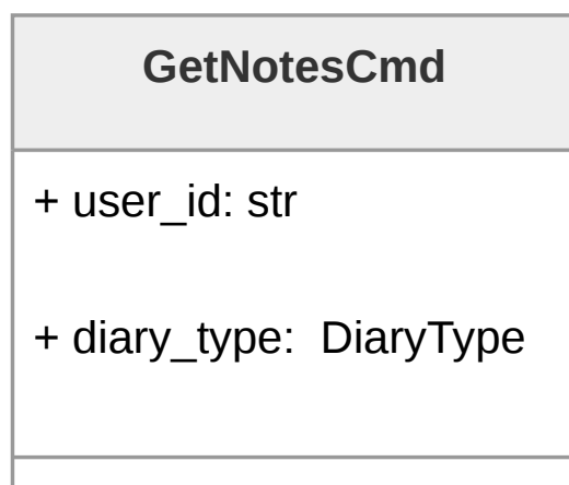
Figura 146: Diagramma della classe GetNotesCmd
