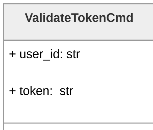
Figura 153: Diagramma della classe ValidateTokenCmd
