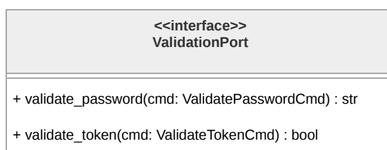
Figura 162: Diagramma dell'interfaccia ValidationPort
