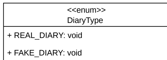
Figura 142: Diagramma dell'enumerazione DiaryType
