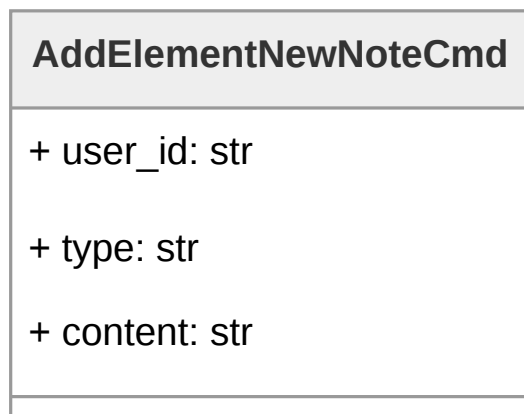
Figura 147: Diagramma della classe AddElementNewNoteCmd
