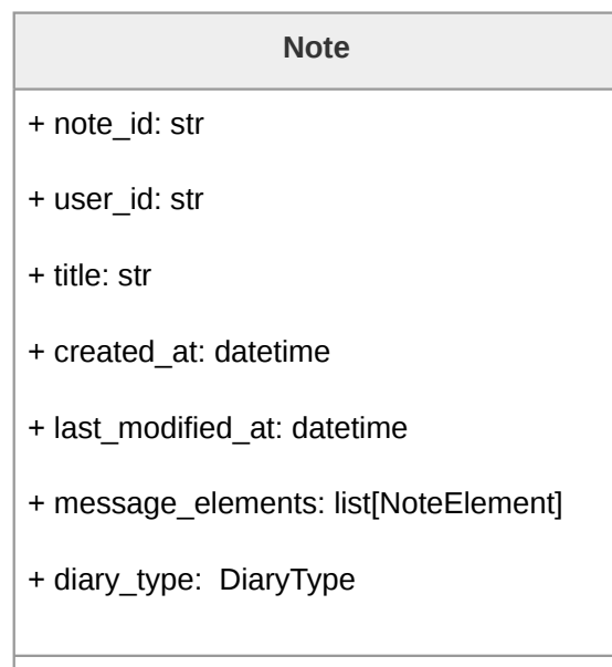
Figura 143: Diagramma della classe Note
