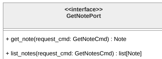
Figura 156: Diagramma dell'interfaccia GetNotePort
