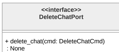
Figura 188: Diagramma dell'interfaccia DeleteChatPort
