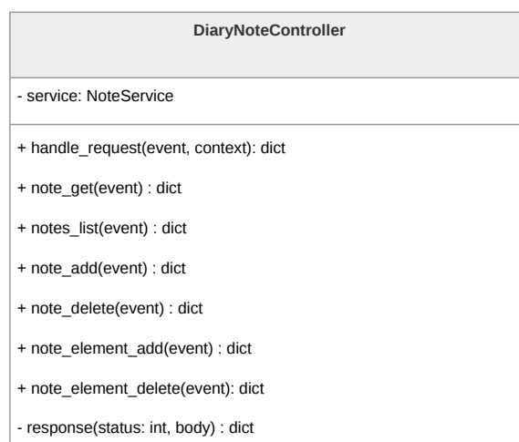
Figura 174: Diagramma della classe DiaryNoteController
