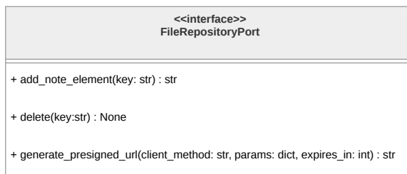
Figura 165: Diagramma dell'interfaccia FileRepositoryPort
