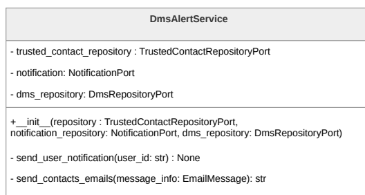
Figura 221: Diagramma della classe DmsAlertService
