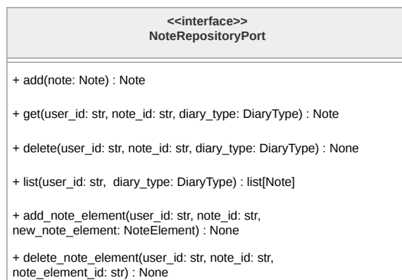
Figura 164: Diagramma dell'interfaccia NoteRepositoryPort
