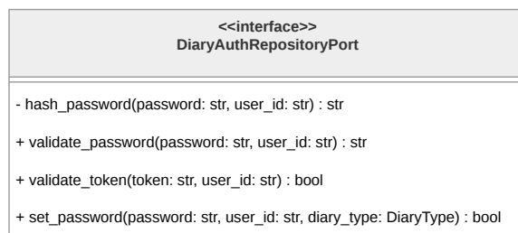
Figura 166: Diagramma dell'interfaccia DiaryAuthRepositoryPort
