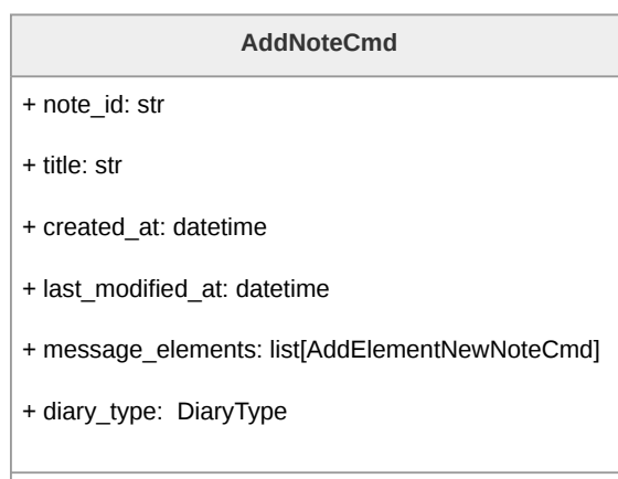
Figura 148: Diagramma della classe AddNoteCmd
