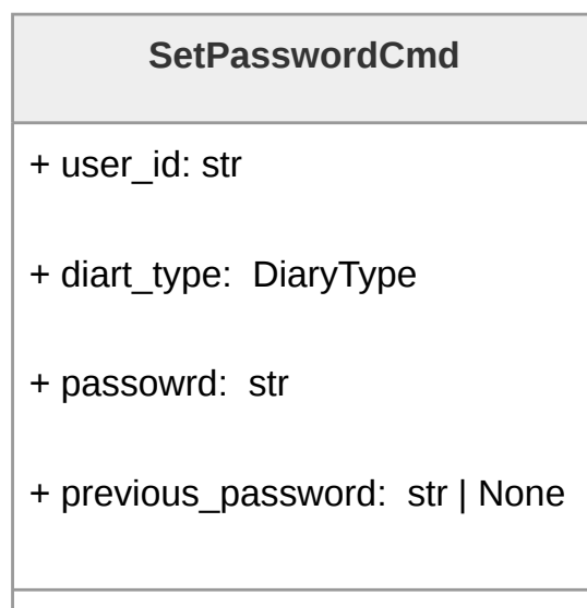
Figura 154: Diagramma della classe SetPasswordCmd
