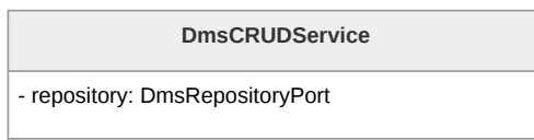
Figura 220: Diagramma della classe DmsCRUDService
