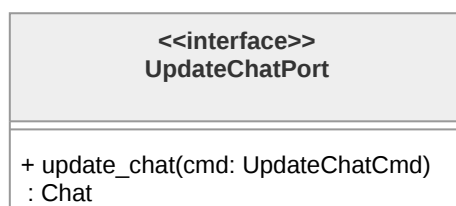
Figura 187: Diagramma dell'interfaccia UpdateChatPort
