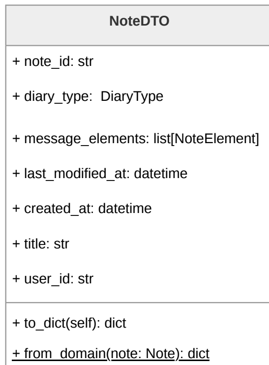
Figura 173: Diagramma della classe NoteDTO
