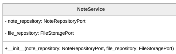
Figura 167: Diagramma della classe NoteService
