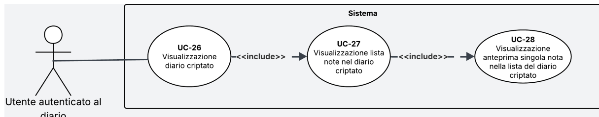
Figura 16: Diagramma del caso d'uso UC-26
