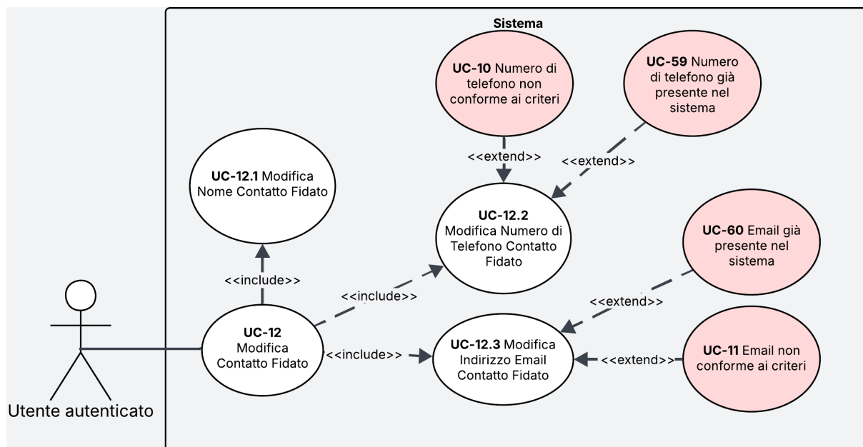
Figura 9: Diagramma del caso d'uso UC-12
