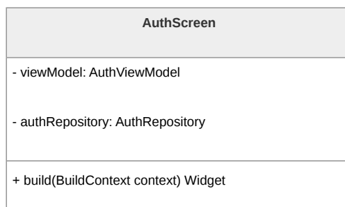
Figura 2: Diagramma della classe AuthScreen
