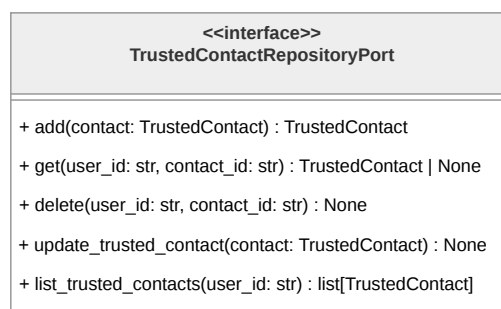
Figura 157: Diagramma della classe TrustedContactRepositoryPort
