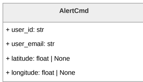
Figura 141: Diagramma della classe AlertCmd
