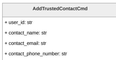
Figura 137: Diagramma della classe AddTrustedContactCmd
