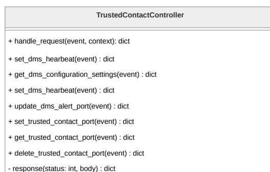
Figura 143: Diagramma della classe TrustedContactController
