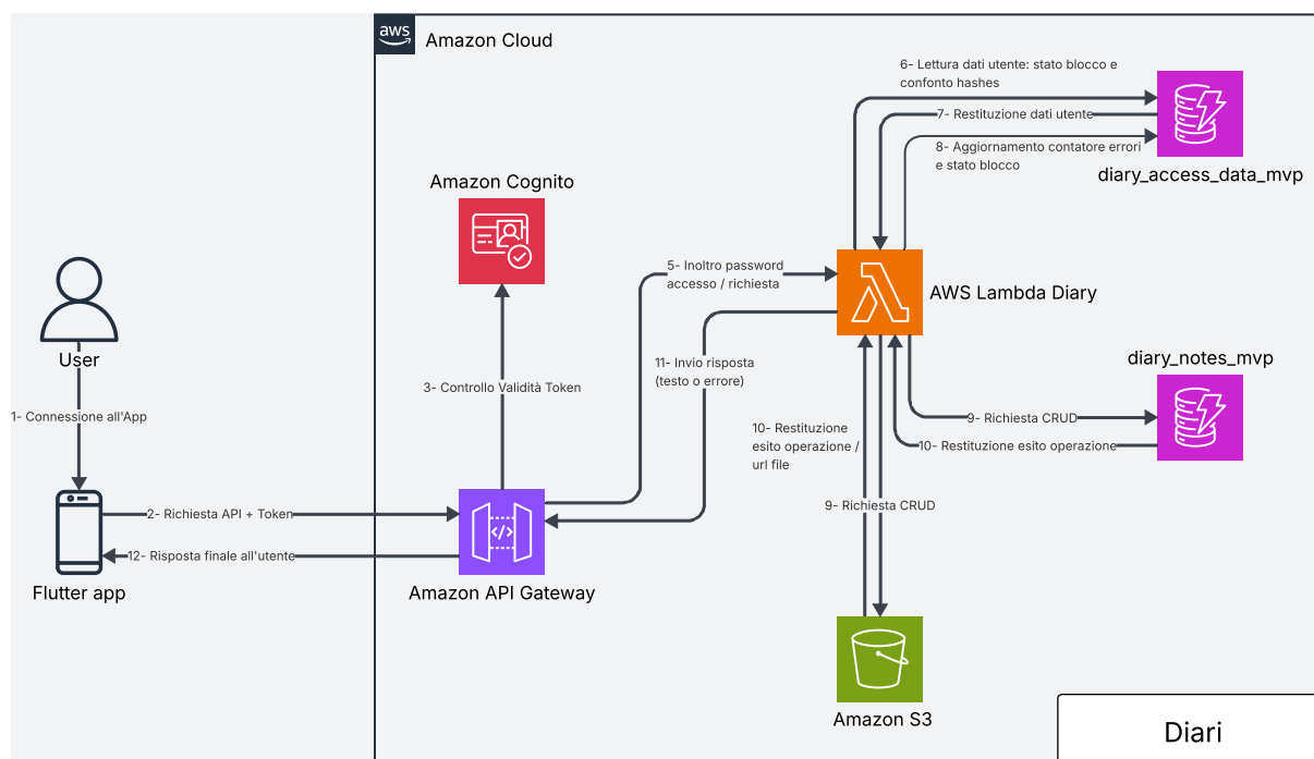
Figura 132: Architettura G diari
