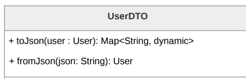
Figura 6: Diagramma della classe UserDTO
