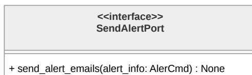
Figura 151: Diagramma della classe SendAlertPort
