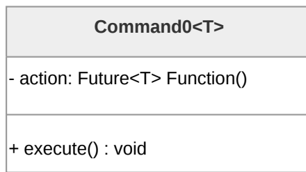
Figura 16: Diagramma della classe Command0<T>
