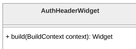
Figura 3: Diagramma della classe AuthHeaderWidget
