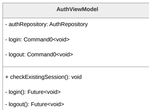
Figura 7: Diagramma della classe AuthViewModel
