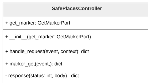
Figura 119: Diagramma della classe SafePlacesController
