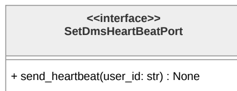
Figura 144: Diagramma della classe SetDmsHeartBeatPort
