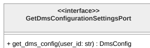
Figura 145: Diagramma della classe GetDmsConfigurationSettingsPort
