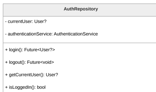
Figura 8: Diagramma della classe AuthRepository
