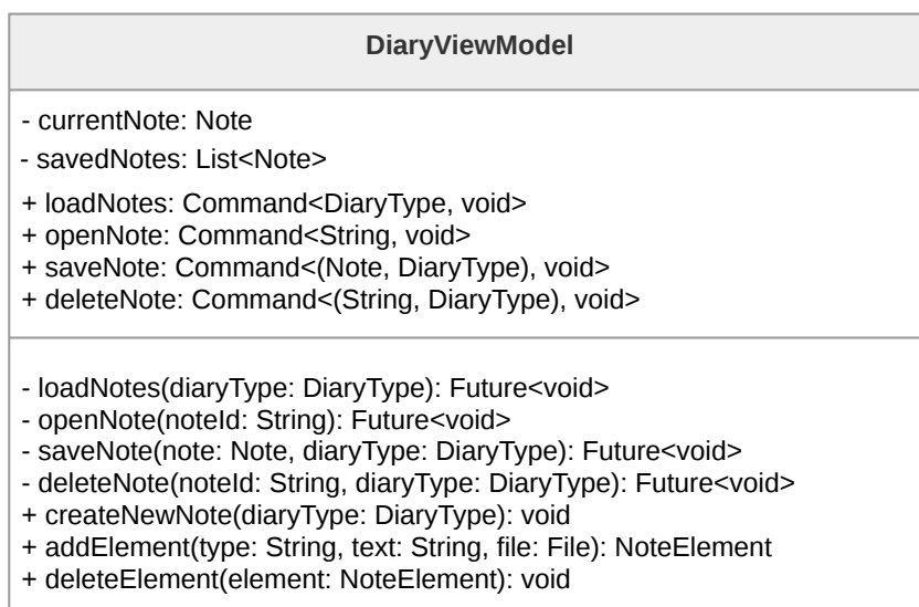
Figura 45: Diagramma della classe DiaryViewModel
