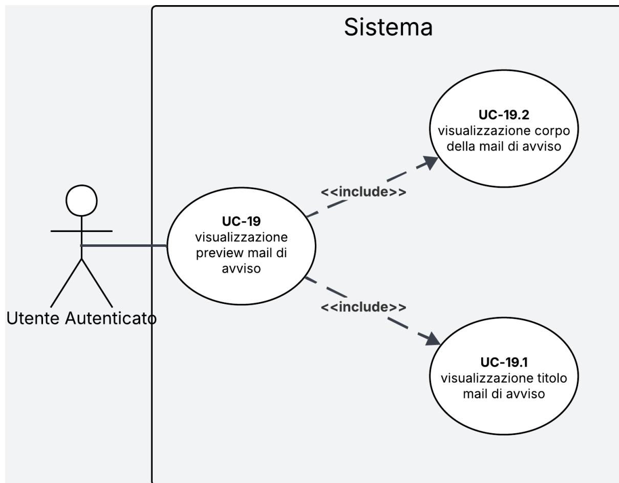
Figura 14: Diagramma del caso d'uso UC-19
