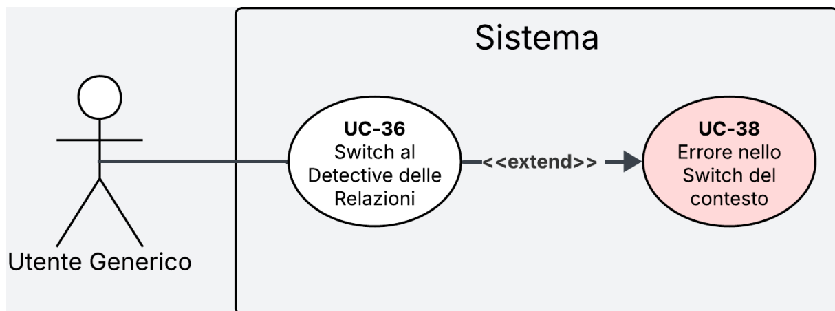
Figura 27: Diagramma del caso d'uso UC-36
