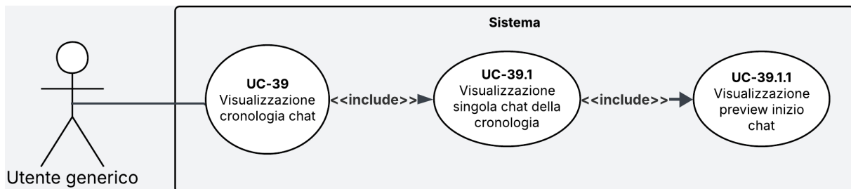
Figura 29: Diagramma del caso d'uso UC-39
