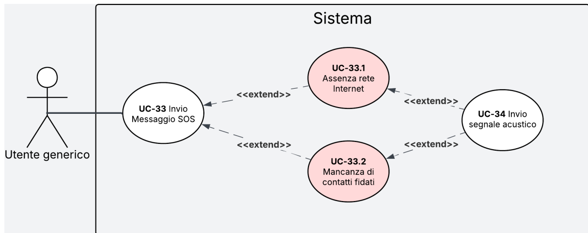
Figura 25: Diagramma del caso d'uso UC-33
