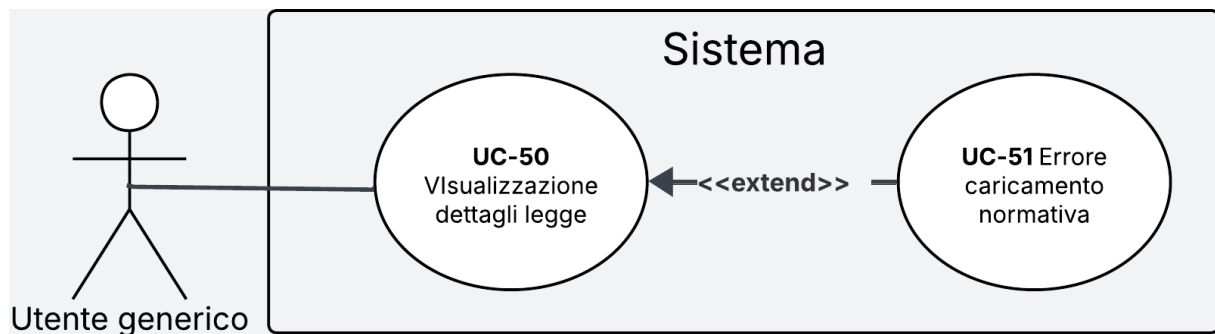
Figura 37: Diagramma del caso d'uso UC-50
