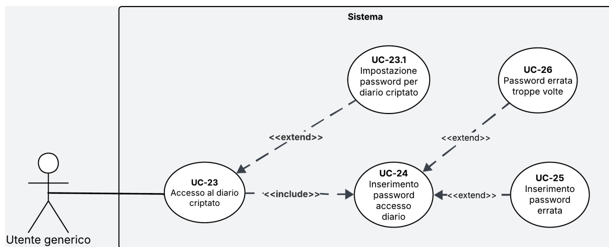
Figura 18: Diagramma del caso d'uso UC-23
