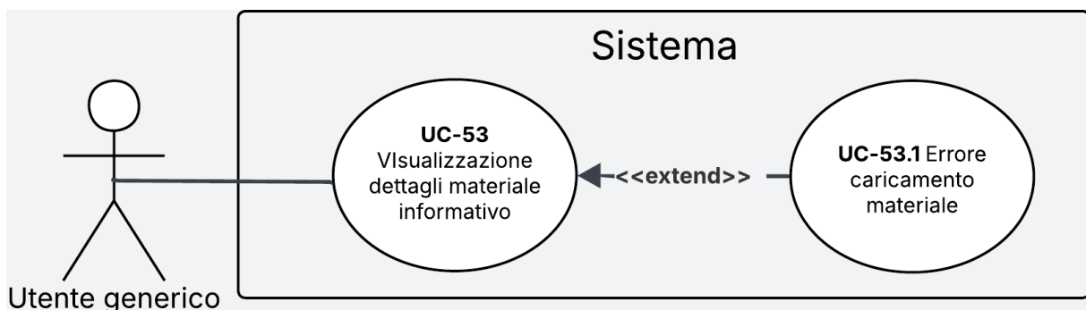
Figura 39: Diagramma del caso d'uso UC-53
