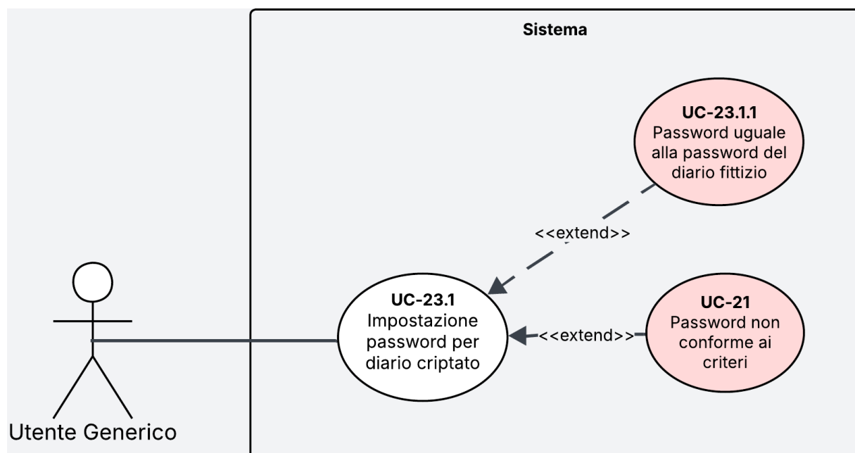
Figura 19: Diagramma del caso d'uso UC-23.1
