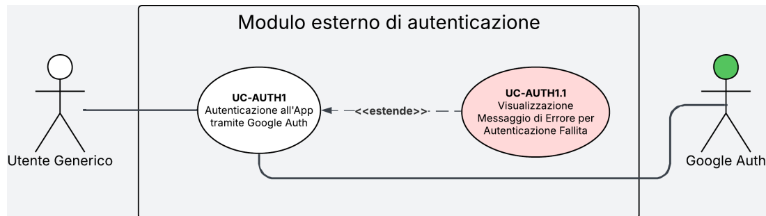
Figura 1: Diagramma dei casi d'uso UC-AUTH1 e UC-AUTH1.1
