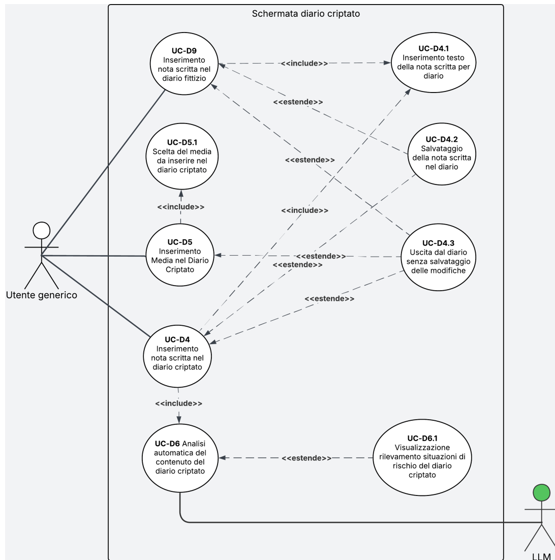
Figura 9: Diagramma dei casi d'uso UC-D4, UC-D5, UC-D6, UC-D9 e i loro relativi casi d'uso che da loro derivano
