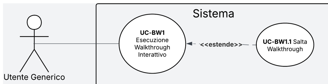
Figura 2: Diagramma del caso d'uso UC-BW1
