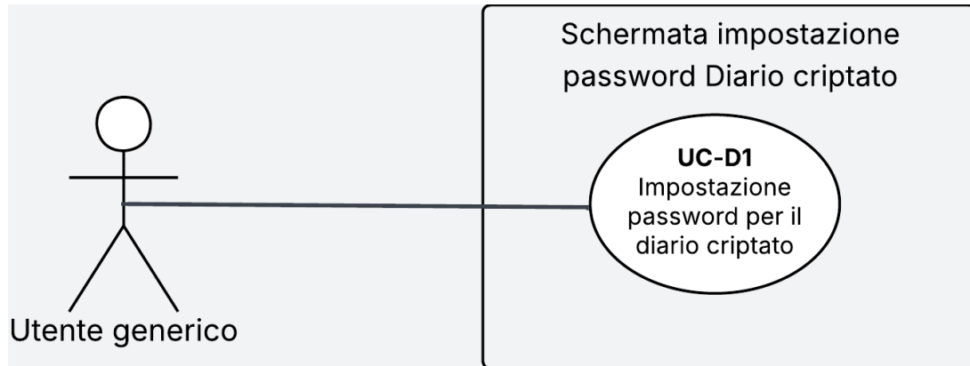
Figura 6: Diagramma del caso d'uso UC-D1
