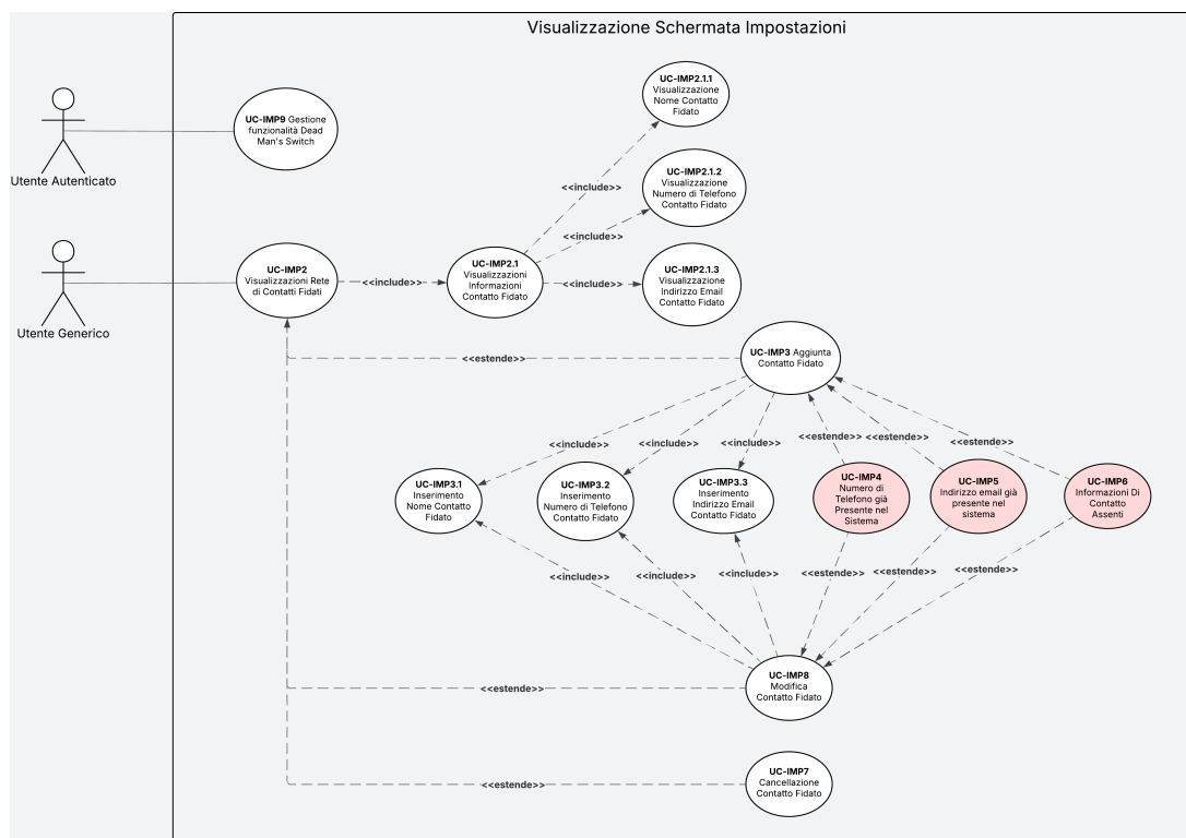
Figura 5: Diagramma dei casi d'uso compresi da UC-IMP1
