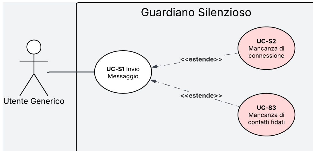
Figura 12: Diagramma del caso d'uso UC-S1 con UC-S2 e UC-S3
