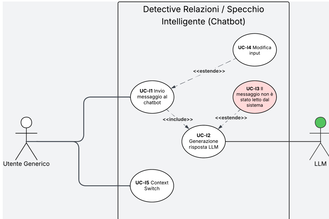
Figura 13: Diagramma Dei casi d'uso UC-I
