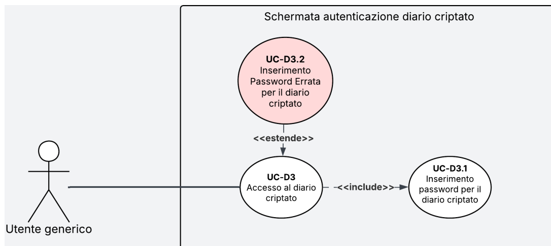
Figura 8: Diagramma del caso d'uso UC-D3
