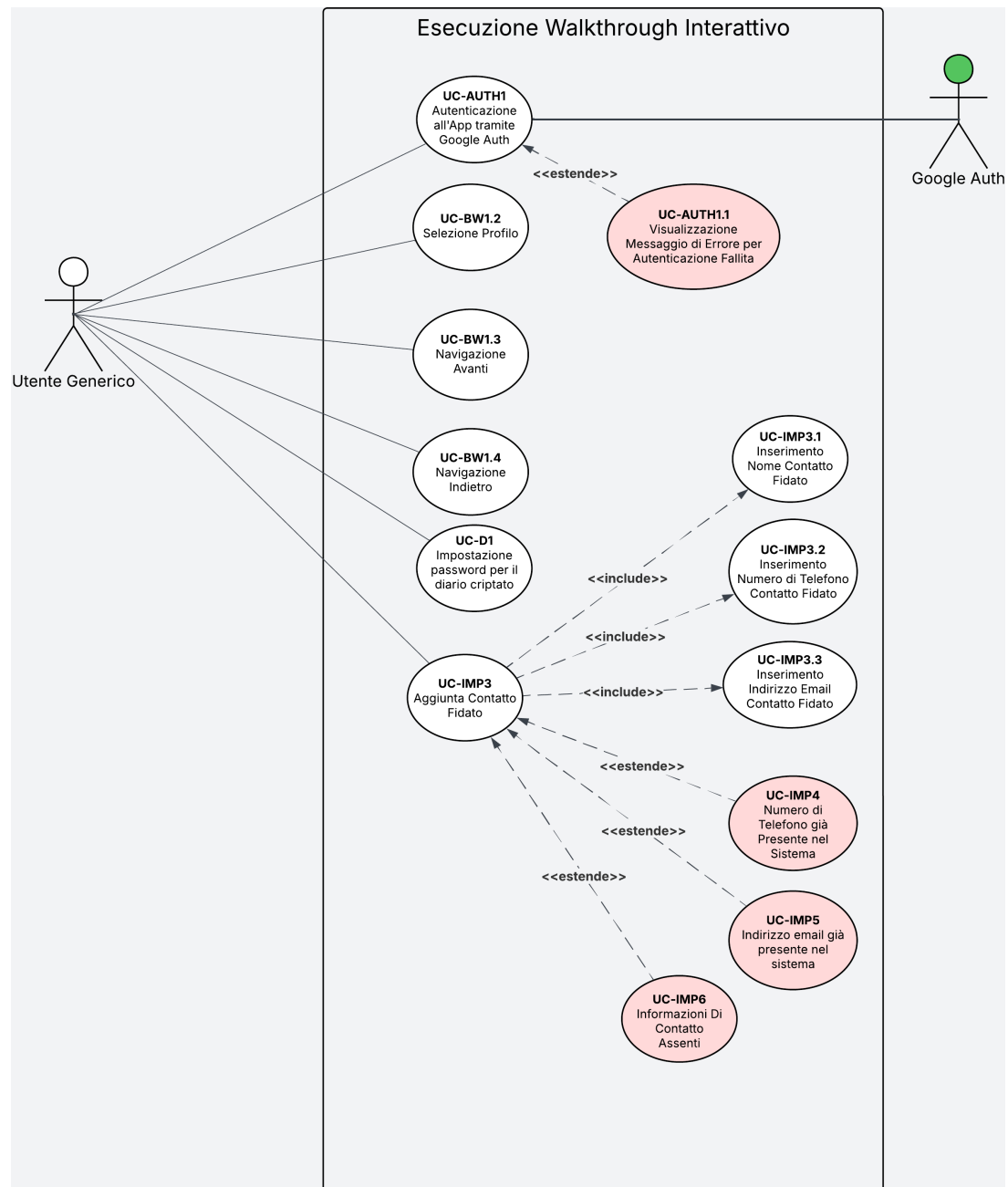
Figura 3: Diagramma dei casi d'uso inclusi ed estesi da UC-BW1
