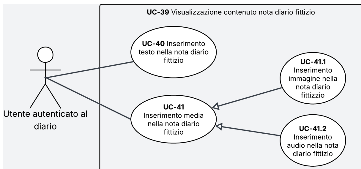
Figura 21: Diagramma dei casi d'uso UC-40, UC-41, UC-41.1 e UC-41.2
