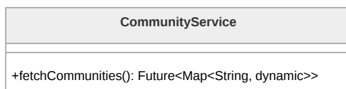
Figura 92: Diagramma della classe CommunityService
