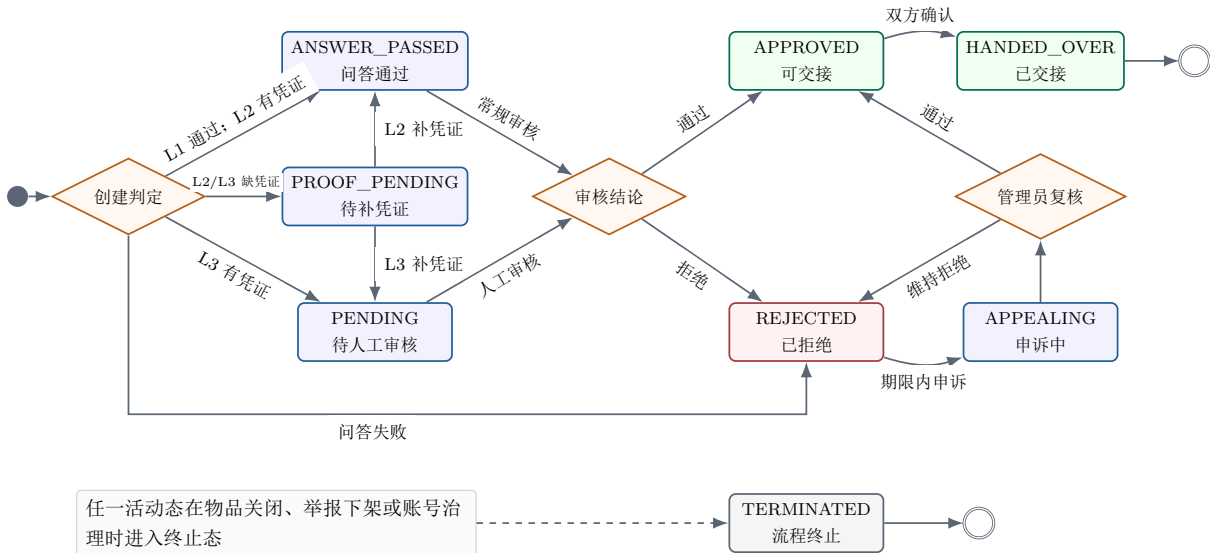
图 4: 认领请求状态图
