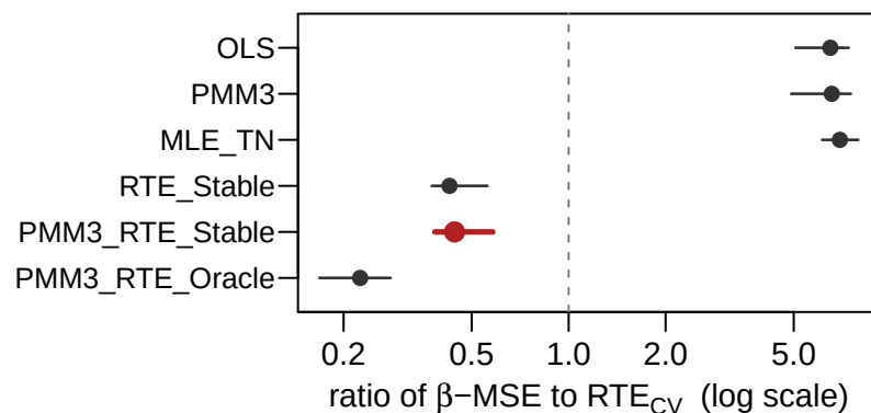
normal: n = 100, \rho = 0.9
