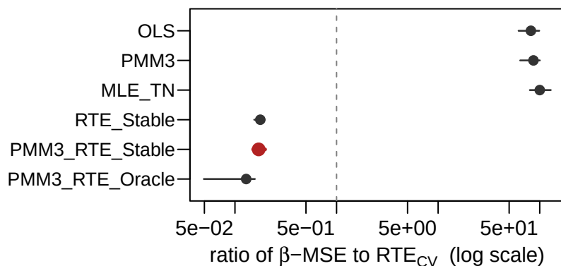
normal: n = 100, \rho = 0.99
