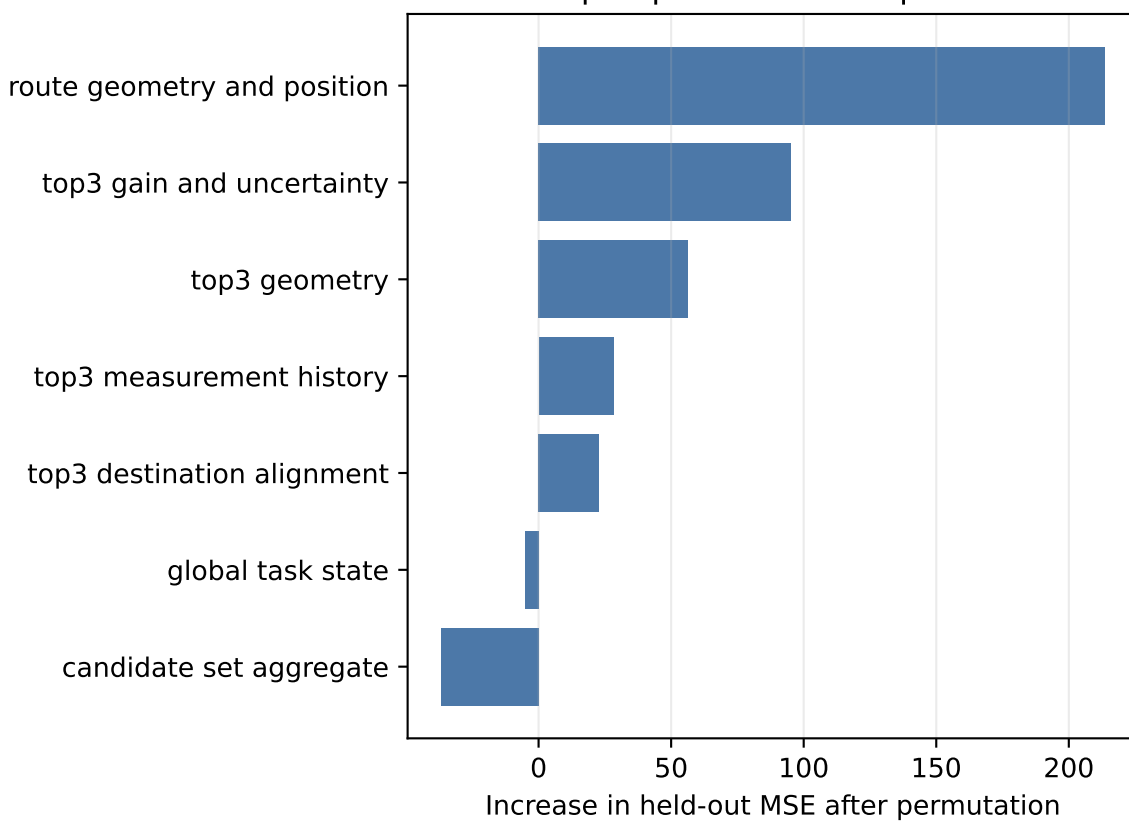
Grouped permutation importance
