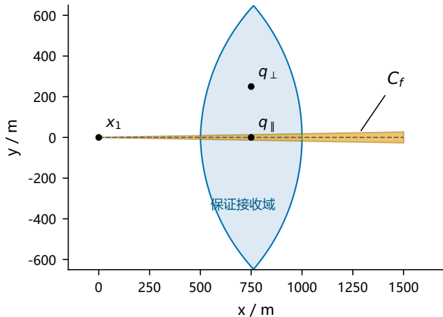
(a) 首测源域与充分安全测点域
