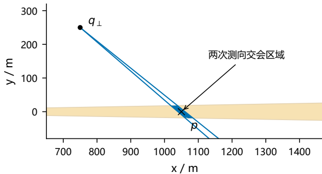
(b) 横向基线的交会示意
