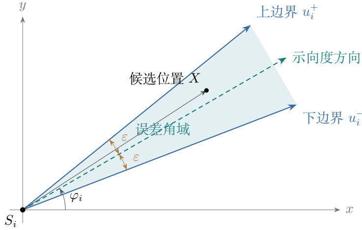
图 1 单次测向的误差角域。为便于辨认，图中误差角作放大示意；模型计算仍取半张角 \varepsilon = 1^\circ 。
