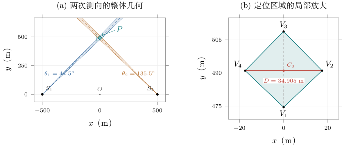
图 2 两次测向的角域交会与定位区域。采用第 5.3 节算例数据，边界角按真实的 \pm 1^\circ 绘制；两幅子图各自保持等比例坐标，右图为交会区域放大。
