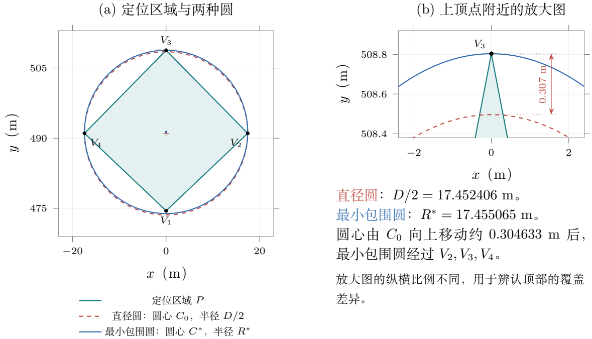
图 3 直径圆覆盖失败与最小包围圆的修正。红色虚线圆在上顶点 V_3 处留下约 0.307 \text{ m} 的覆盖缺口; 蓝色实线圆覆盖全部顶点。左图按等比例绘制, 右图单独放大顶部差异。
