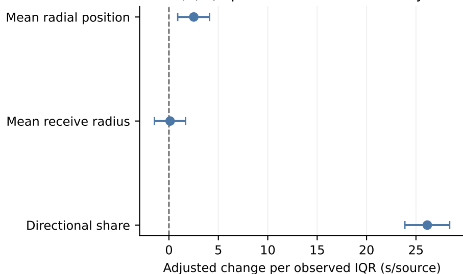
(d) Q4 partial scenario sensitivity
