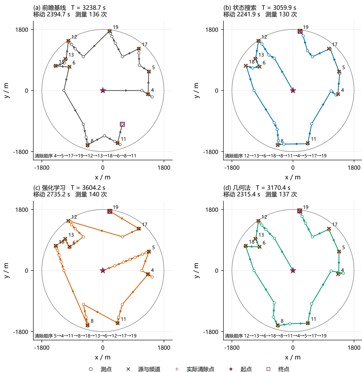
图 9: PPO 最大退化场景 800081。该例主要额外代价来自移动，PPO 较基线慢 365.45 s；此例不表示总体发生频率。
