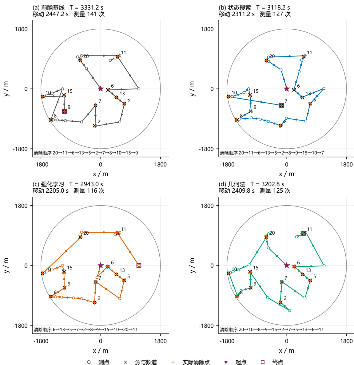
图 7: 基线中位耗时附近场景 800035 的四方法真实轨迹。统一坐标比例, 箭头表示移动方向, 源旁数字为频道, 面板底部列出实际清除顺序。同坐标多次测量合并显示位置, 但测量次数保留原始计数。
