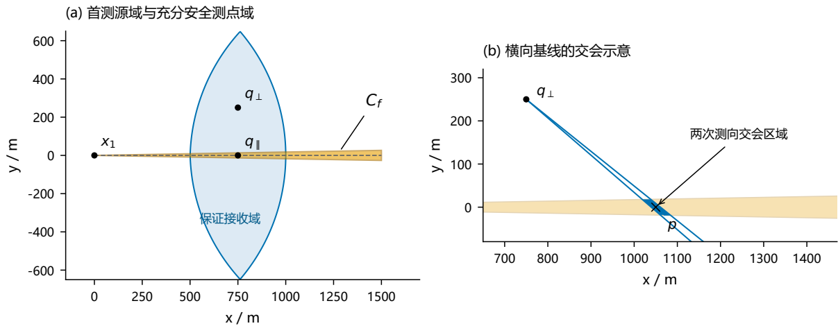
图 2: 首测可行域及横向交会的解析示意。半角采用 1.005^\circ ，蓝色测点域由三角外包构造，属于充分保证接收域；示意源 p 仅用于解释交会几何，不作为规划输入。右图展示另一比例下的局部几何，不能作为算法性能比较。
