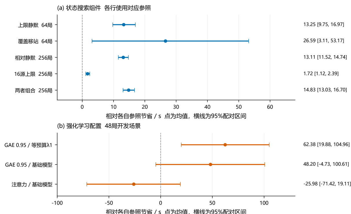
图 6: 核心组件及训练配置的消融结果。正值表示节省，各行以各自冻结参照计算；上部的 64 局和 256 局来自不同实验批次，下部为 48 局开发结果。不同批次收益不作相加。
