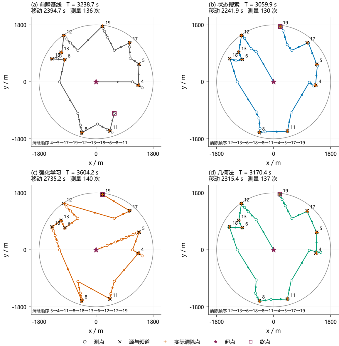
图 9: PPO 最大退化场景 800081。该例主要额外代价来自移动，PPO 较基线慢 365.45 s；此例不表示总体发生频率。
