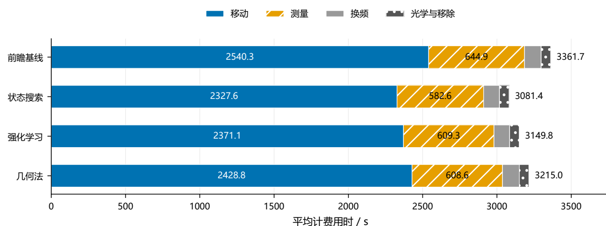
图 5: 首版随机集的平均费用分解。分项之和等于整局计费用时; 移动是主要成本, 但扫描与换频的节省同样影响总结果。
