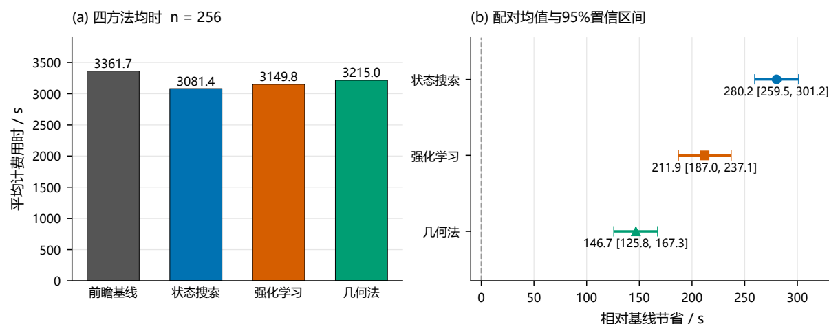
图 4: 首版四方法在同一 256 随机场景上的均时与配对节省。右图为相对前瞻基线的 95% 配对 bootstrap 区间, 不能当作左图各均时的区间。
