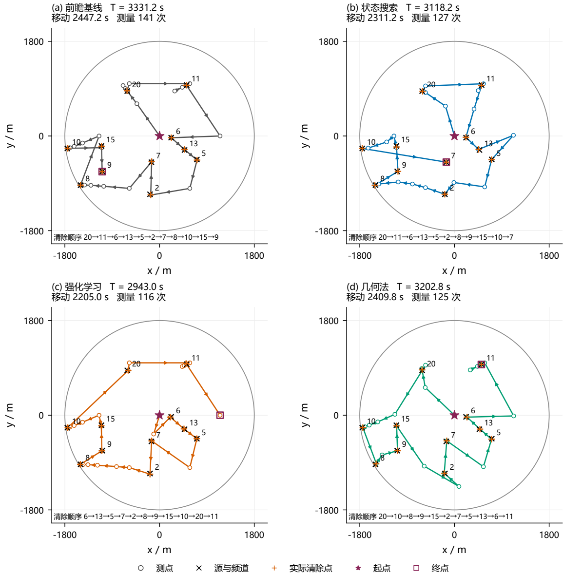
图 7: 基线中位耗时附近场景 800035 的四方法真实轨迹。统一坐标比例, 箭头表示移动方向, 源旁数字为频道, 面板底部列出实际清除顺序。同坐标多次测量合并显示位置, 但测量次数保留原始计数。
