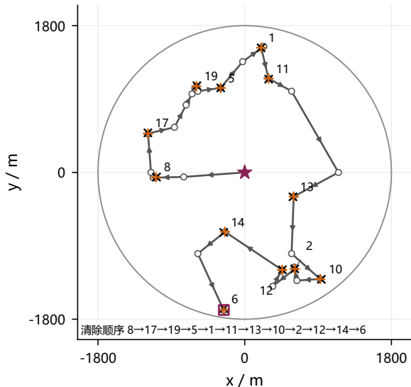
(c) 强化学习 T = 2843.1 s 移动 2094.1 s 测量 117 次
