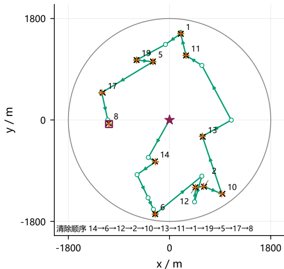
(d) 几何法 T = 2935.5 s 移动 2156.5 s 测量 121 次
