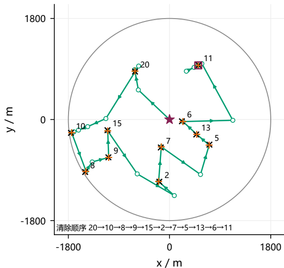
(d) 几何法 T = 3202.8\text{ s} 移动 2409.8 s 测量 125 次
