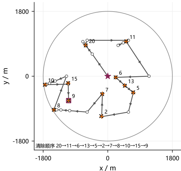
(c) 强化学习 T = 2943.0\text{ s} 移动 2205.0 s 测量 116 次
