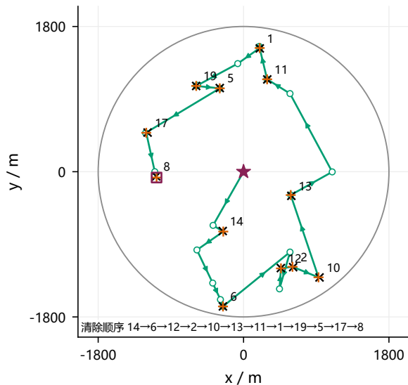
(d) 几何法 T = 2935.5\text{ s} 移动 2156.5 s 测量 121 次
