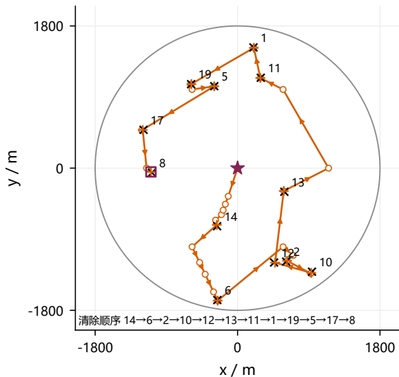
(c) 强化学习 T = 2843.1\text{ s} 移动 2094.1 s 测量 117 次
