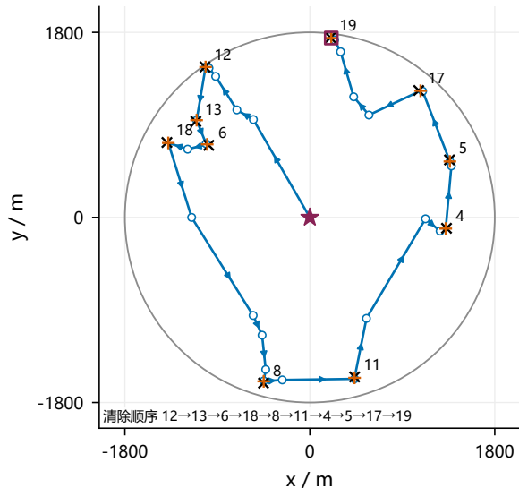
(d) 几何法 T = 3170.4\text{ s} 移动 2315.4 s 测量 137 次
