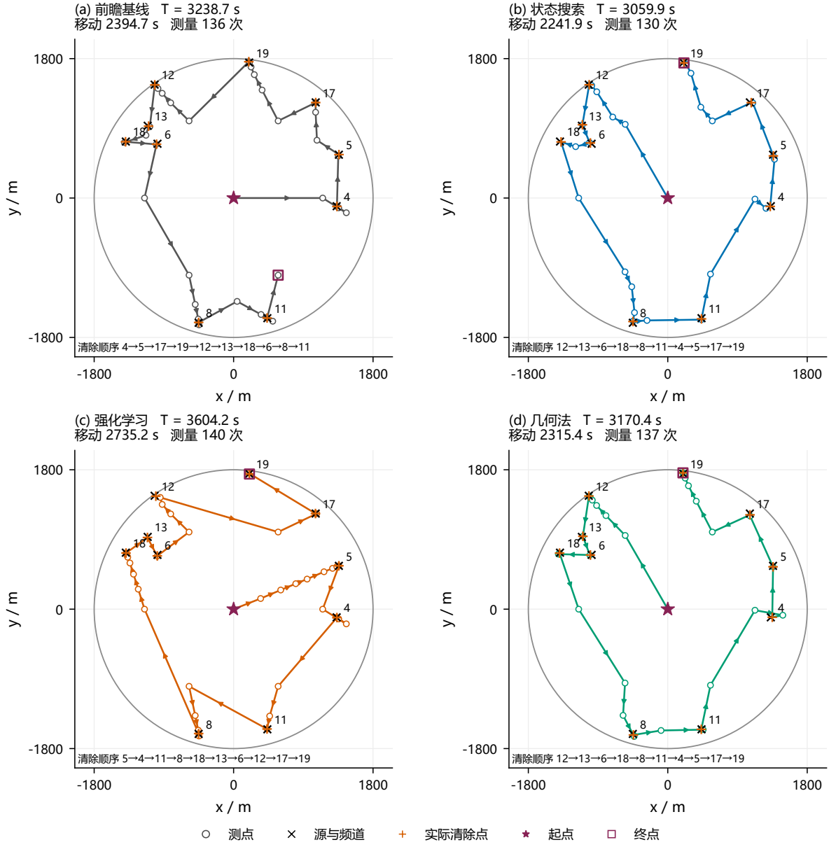
图 8 PPO 最大退化场景 800081。该例主要额外代价来自移动，PPO 较基线慢 365.45\text{ s} ；此例不表示总体发生频率。
