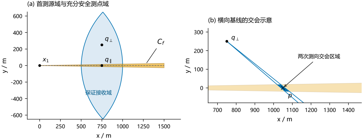
图 1 首测可行域及横向交会的解析示意。半角采用 1.005^\circ ，蓝色测点域由三角外包构造，属于充分保证接收域；示意源 p 仅用于解释交会几何，不作为规划输入。右图展示另一比例下的局部几何，不能作为算法性能比较。
