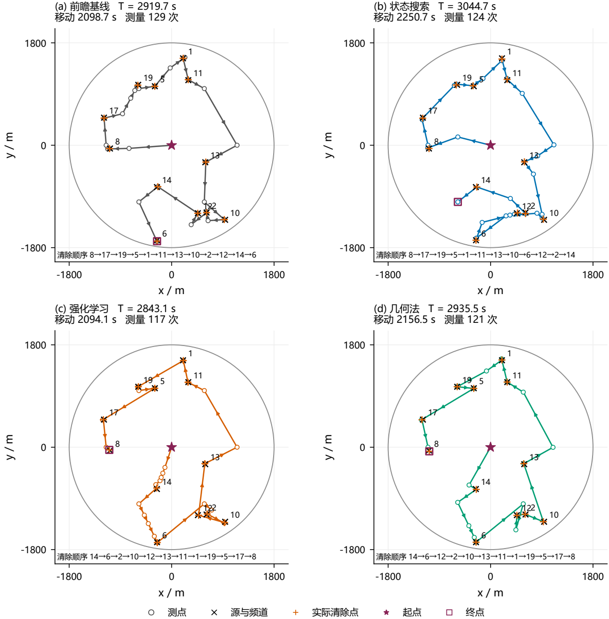
图 7 状态搜索最大退化场景 800015。状态搜索虽减少检测，却因移动增长而较基线慢 125.08\text{ s} ；此例为事后诊断选择。
