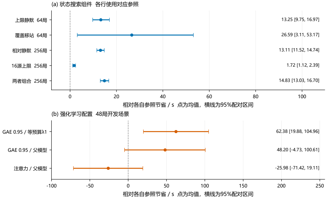
图 5 核心组件及训练配置的消融结果。正值表示节省，各行以各自冻结参照计算；上部的 64 局和 256 局来自不同实验批次，下部为 48 局开发结果。不同批次收益不作相加。
