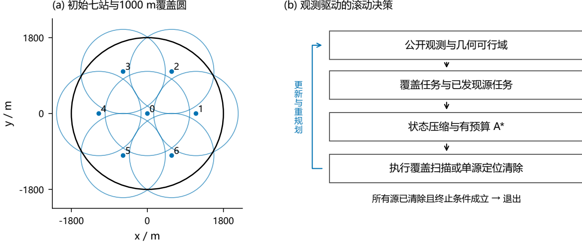
图 2 初始发现覆盖与滚动决策框架。七个 1000 m 接收保证圆覆盖半径 1800 m 场地；未来站移动后仍需重新通过全域覆盖核验。
