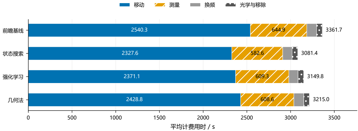
图 4 首版随机集的平均费用分解。分项之和等于整局计费用时；移动是主要成本，但扫描与换频的节省同样影响总结果。
