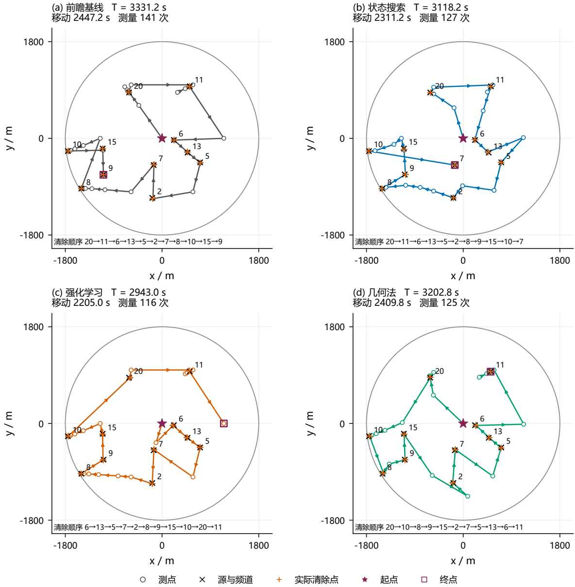
图 6 基线中位耗时附近场景 800035 的四方法真实轨迹。统一坐标比例，箭头表示移动方向，源旁数字为频道，面板底部列出实际清除顺序。同坐标多次测量合并显示位置，但测量次数保留原始计数。
