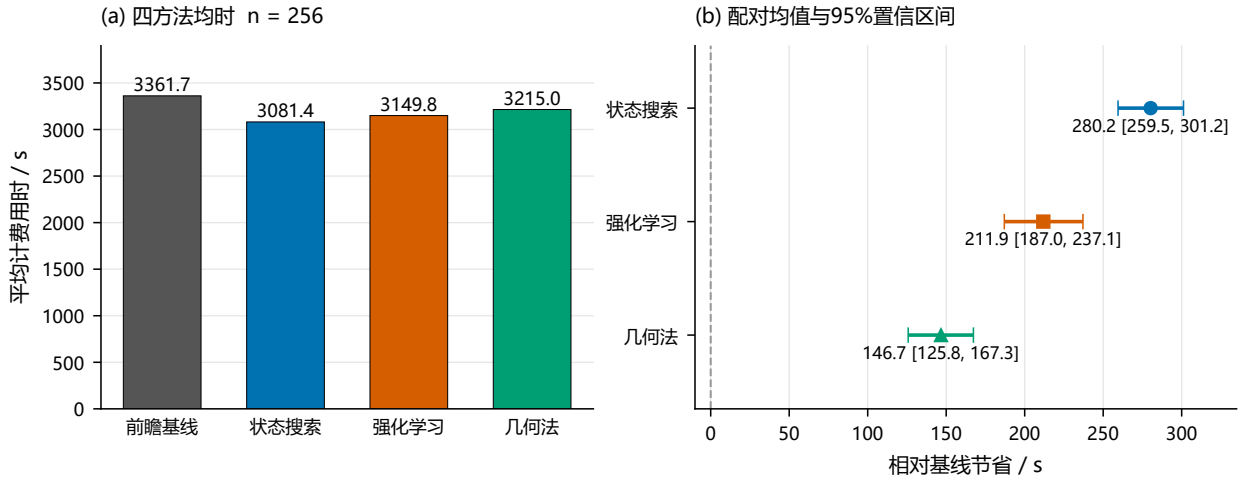
图 3 首版四方法在同一 256 随机场景上的均时与配对节省。右图为相对前瞻基线的 95% 配对 bootstrap 区间，不能当作左图各均时的区间。
