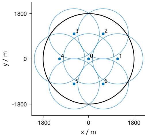
(a) 初始七站与1000 m覆盖圆
