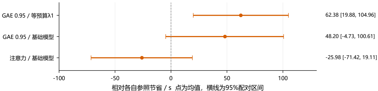
(b) 强化学习配置 48局开发场景
