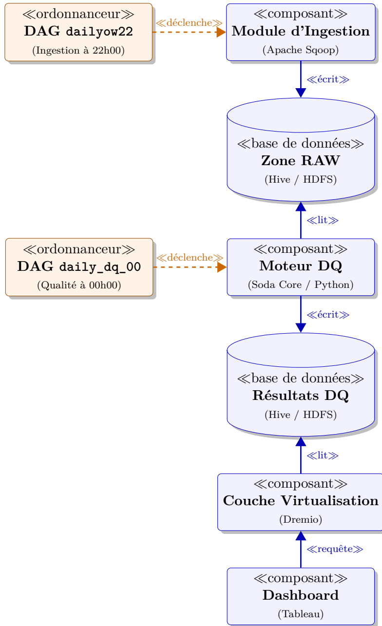
FIGURE 9 – Diagramme de composants logiciels de la solution DQ
