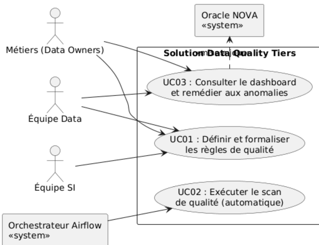
FIGURE 5 – Diagramme global des cas d'utilisation de la solution DQ Tiers
