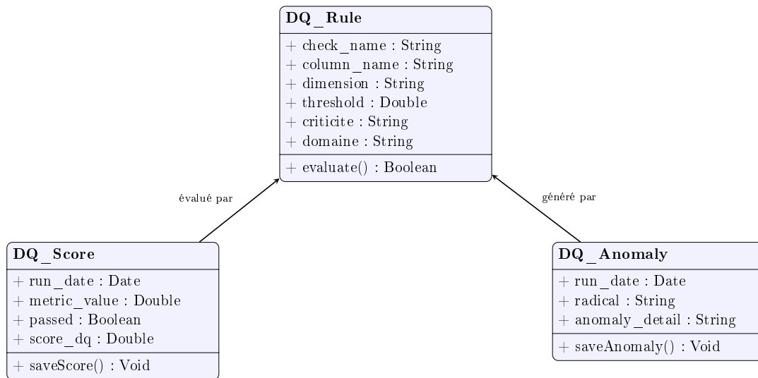
FIGURE 9 – Diagramme de classes des métadonnées de qualité de données
