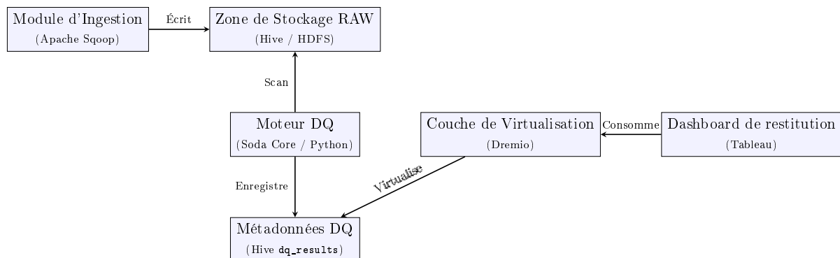
FIGURE 10 – Diagramme de composants logiciels de la solution DQ
