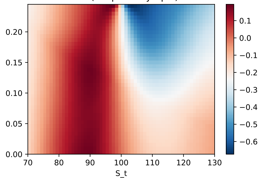
Ecart (deep - analytique)
