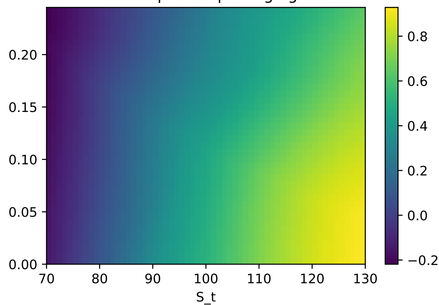
Politique Deep Hedging
