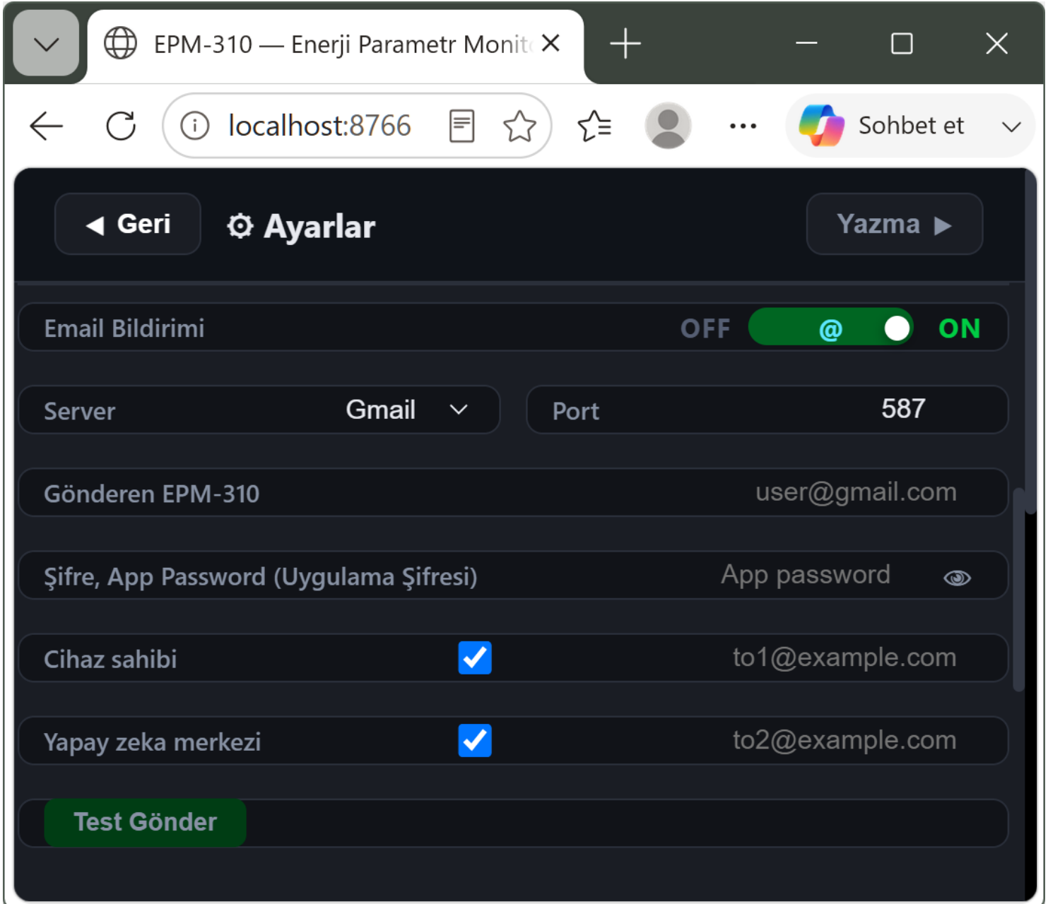
Sek. 7 — Ayarlar sayfası — yapılandırma email Bildirimleri
