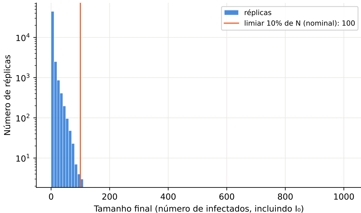
Tamanho final — C3 (vacinação acima do limiar) (n = 48622 réplicas)
