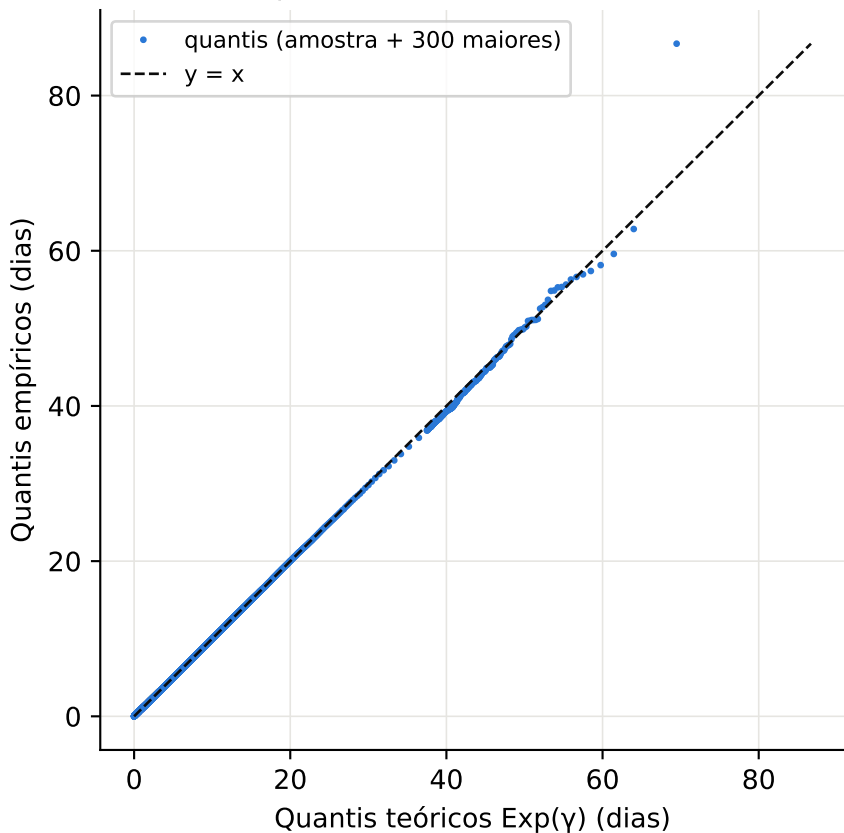
QQ-plot — duração infecciosa (C1)
