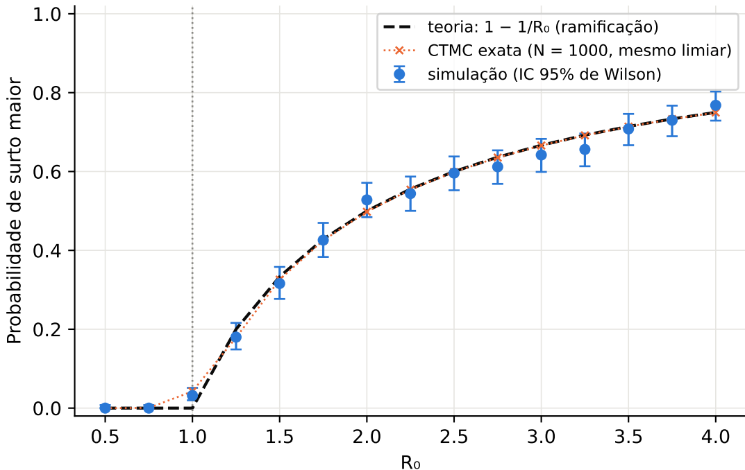
Probabilidade de surto maior \times R_0 ( N = 1000 , I_0 = 1 )
