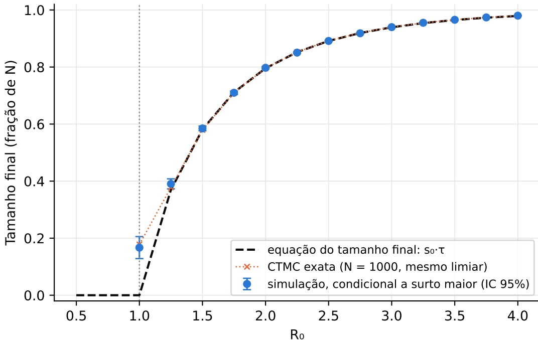
Tamanho final condicional \times R_0 ( N = 1000 , I_0 = 1 )
