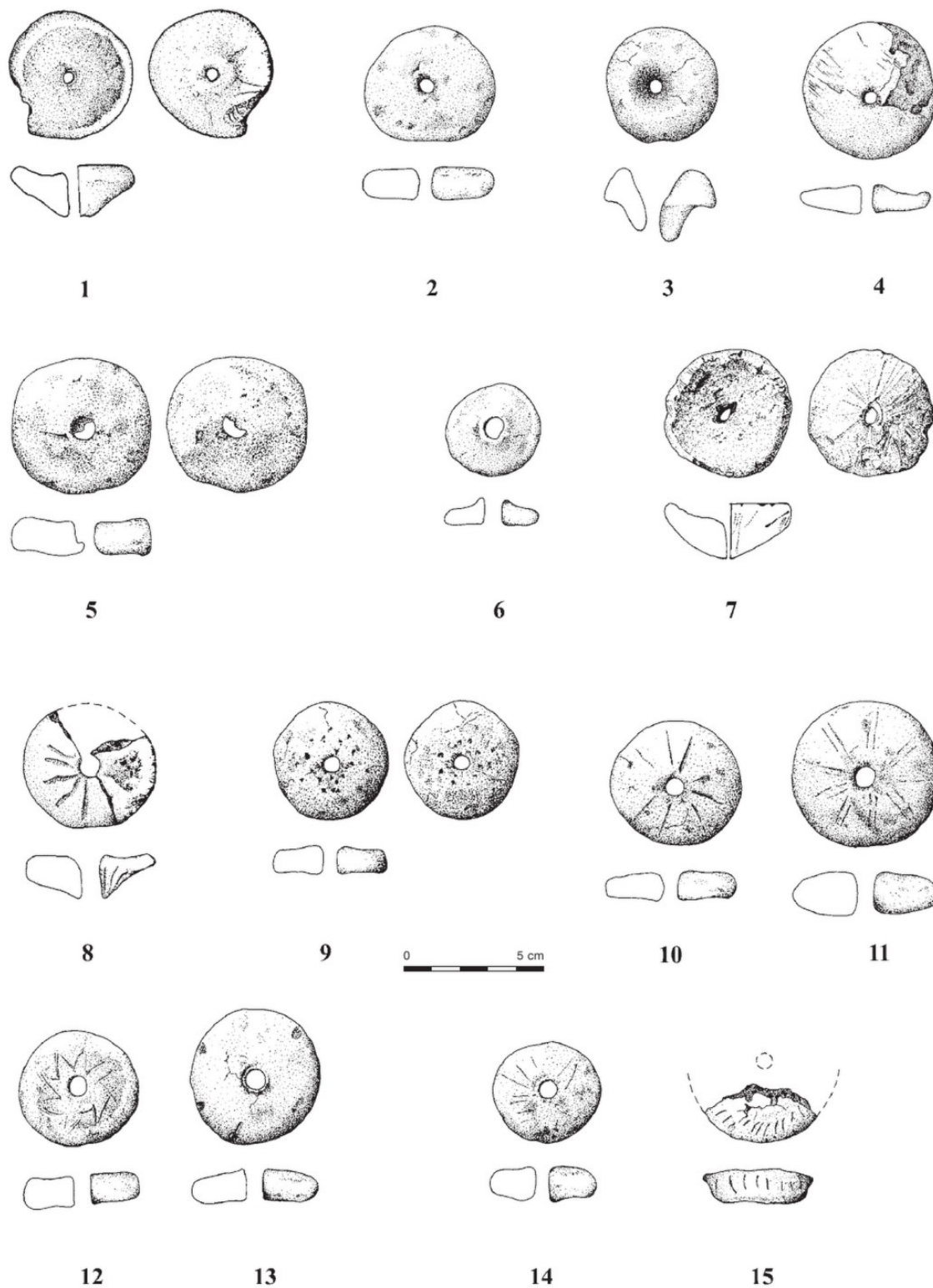
Fig. 7 – Arbon-Bleiche 3 (TG) : caractéristiques de façonnage des fusaïoles. N os 1, 2, 3 et 4 : contours irréguliers et perforations décentrées ; n os 5, 6 et 7 : perforations déformées ; n os 8 à 15 : fusaïoles décorées.
