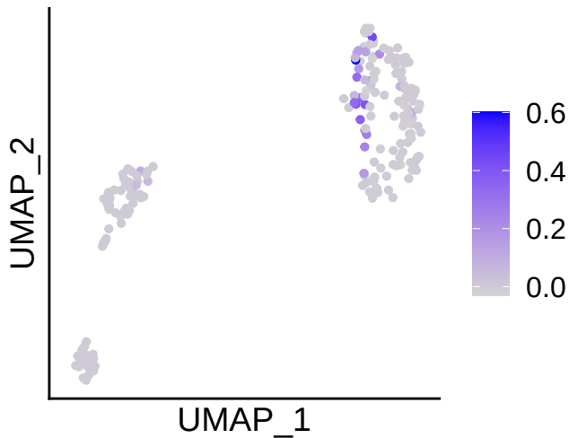
g2m.genes_original
