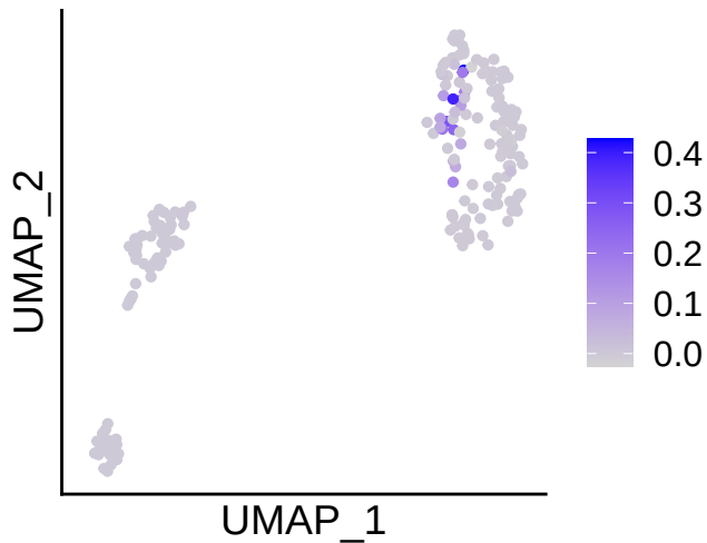
s.genes_original
